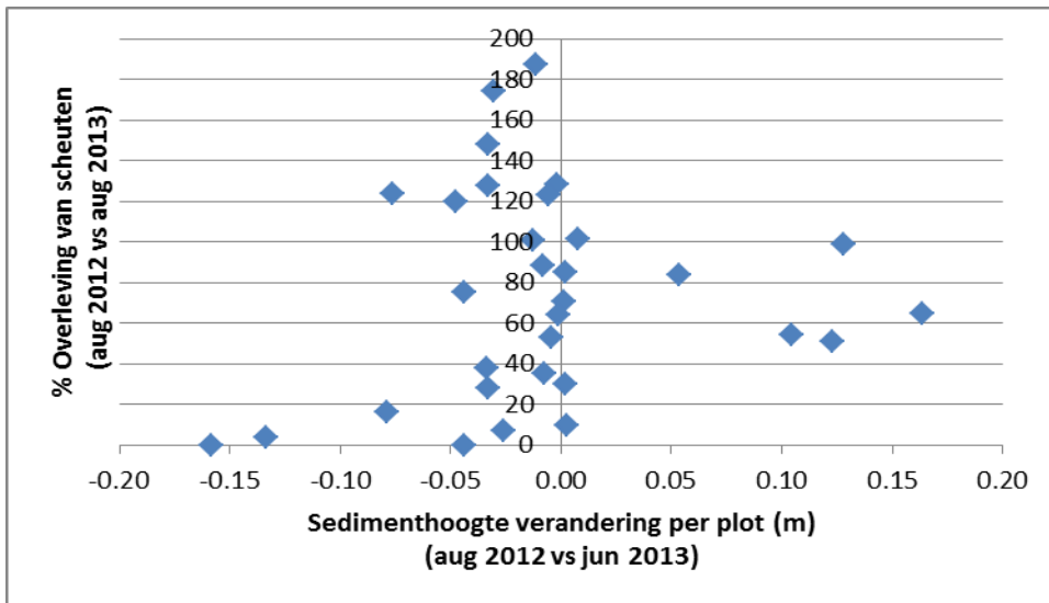
Figuur 50 Erosie/sedimentatie (GNSS) per plot (aug 2012 vs jun 2013) op RH11
