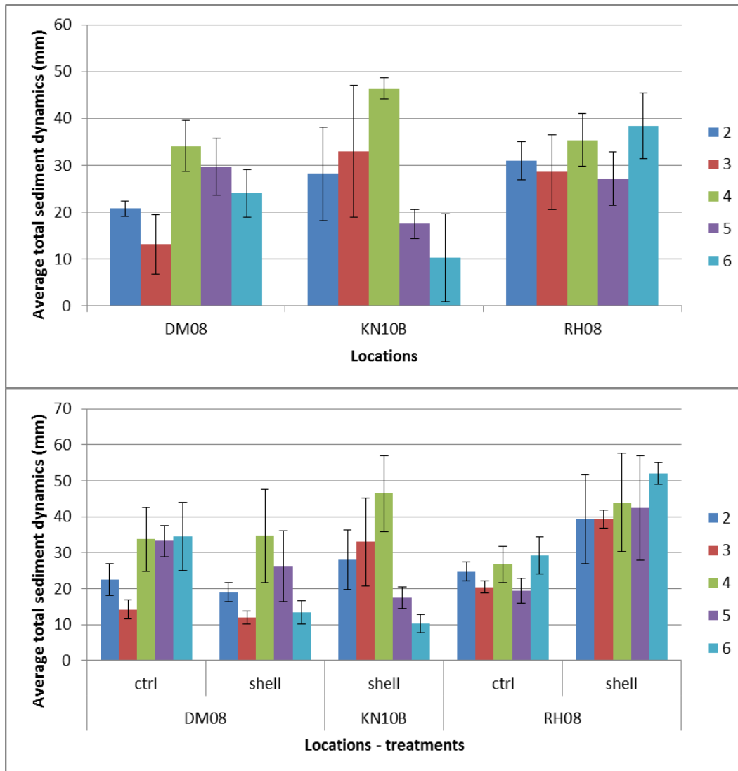
Figuur 48 Totale sedimentdynamiek (=erosie/sedimentatie plus mixing) over de gemeten intervallen per locatie (A, boven) en behandeling (B, onder).
