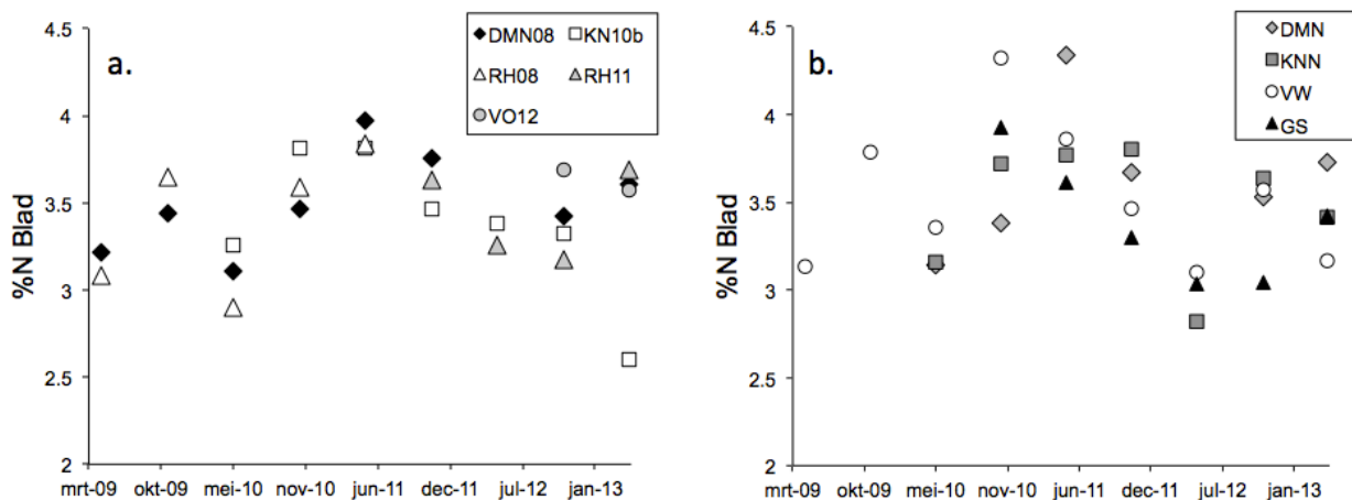
Figuur 24 Stikstof (% N) in blad van a) Transplantatie locaties en b) Natuurlijke populaties
