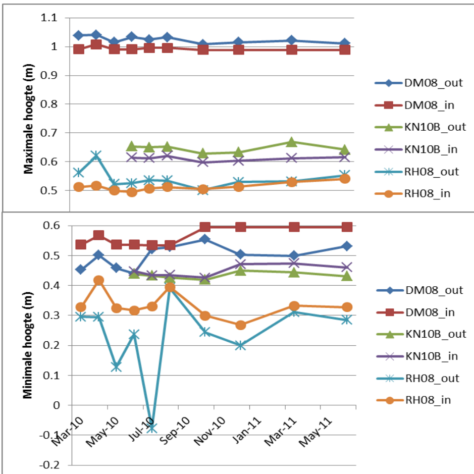
Figuur 44 A) (boven) maximale & B) (onder) minimale hoogteligging (GNSS) van plots over de tijd Onderverdeling in hoogte van zeegrasplaggen (in) en sediment daarbuiten (out).
