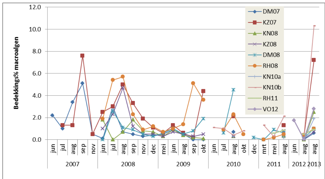
Figuur 38 Bedekkings% macroalgen per mitigatielocatie
