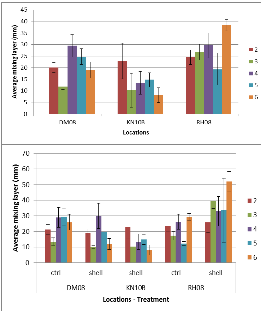
Figuur 47 Dikte van de mixinglaag over de gemeten intervallen per locatie (A, boven) en behandeling (B, onder) Errorbars geven standaardafwijking weer.
