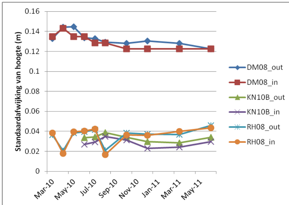
Figuur 45 Variatie in hoogteligging (GNSS) van plots over de tijd uitgedrukt als standaardafwijking
