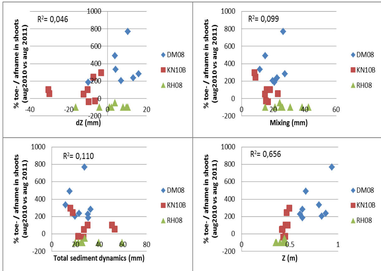
Figuur 49 Sedimentdynamiekparameters en absolute hoogteligging (x-as) uitgezet tegen de procentuele toe- dan wel afname in aantal scheuten in de periode aug 2010 tot aug 2011 (y-as).
