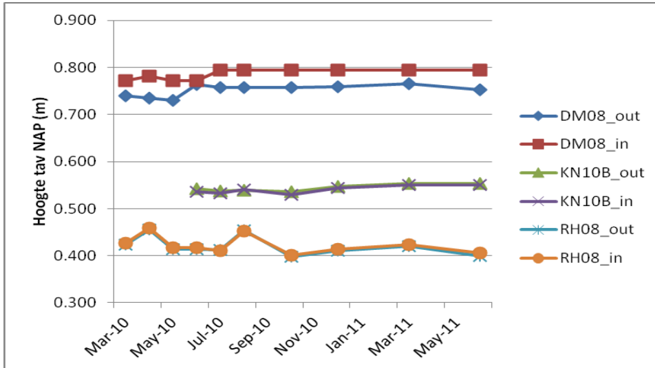
Figuur 43 Gemiddelde hoogteligging (GNSS) van plots over de tijd Onderverdeling in hoogte van zeegrasplaggen (in) en sediment daarbuiten (out).
