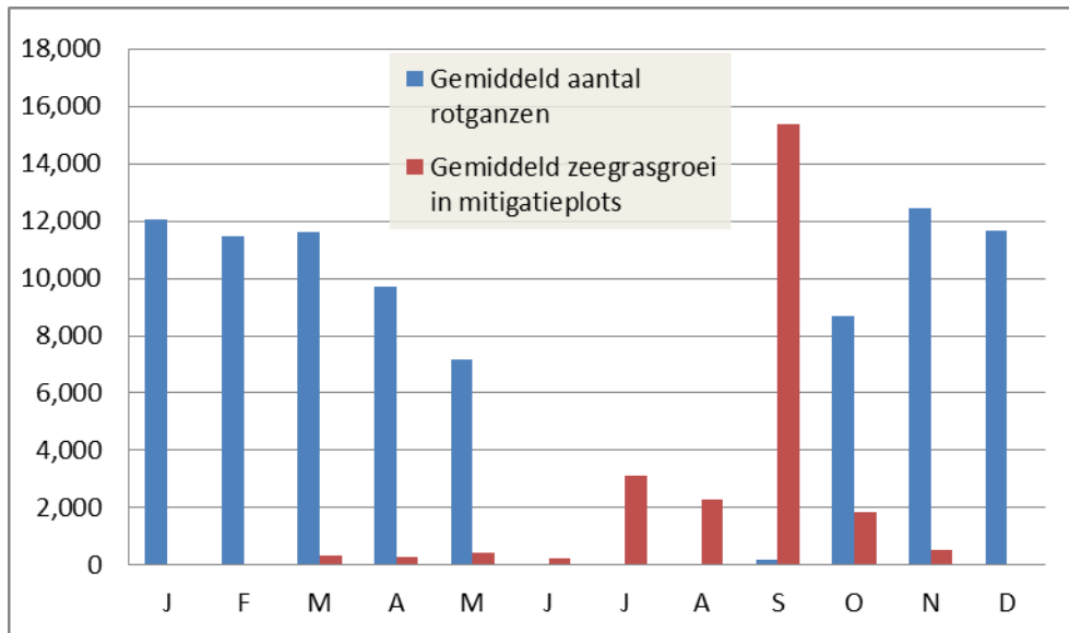
Figuur 39 Gemiddeld aantal rotganzen in Oosterschelde en klein zeegras in mitigatieplots
