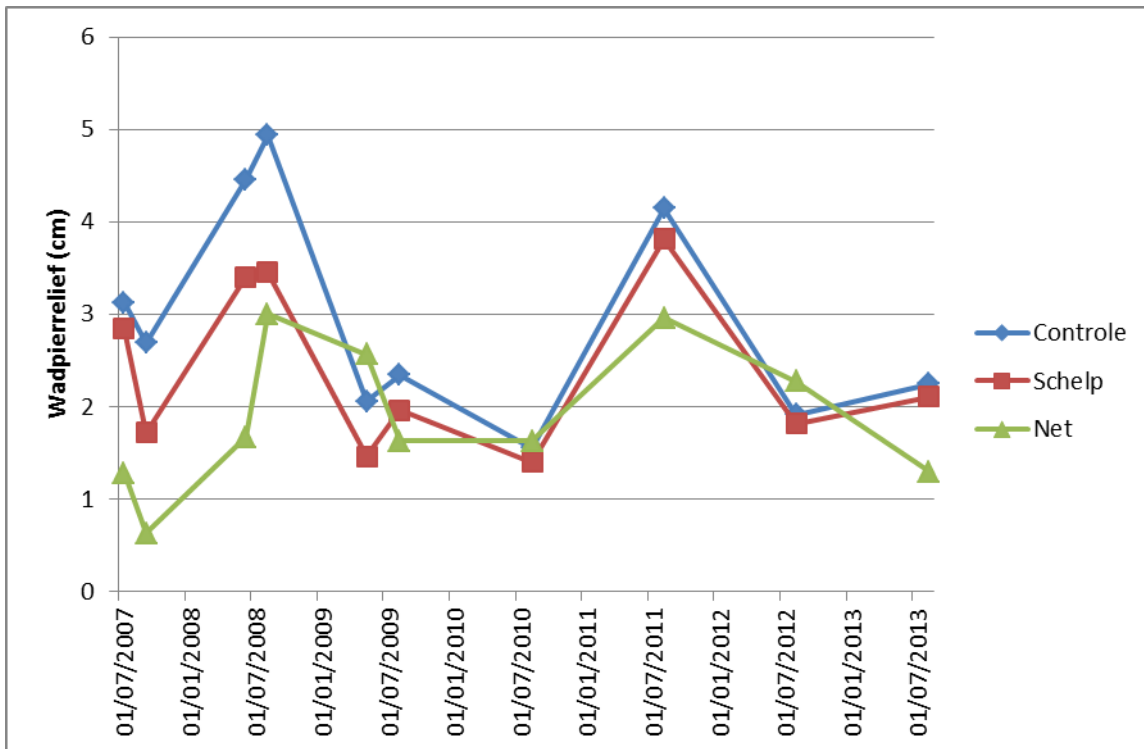
Figuur 34 Gemiddeld wadpierreliëf per behandelingstype
