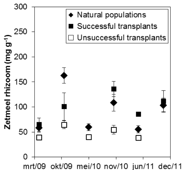
Figuur 25 Zetmeelgehaltes in rhizomen natuurlijke populaties, succesvolle- & niet-succesvolle transplantaties (mg per g gevriesdroogd materiaal)
