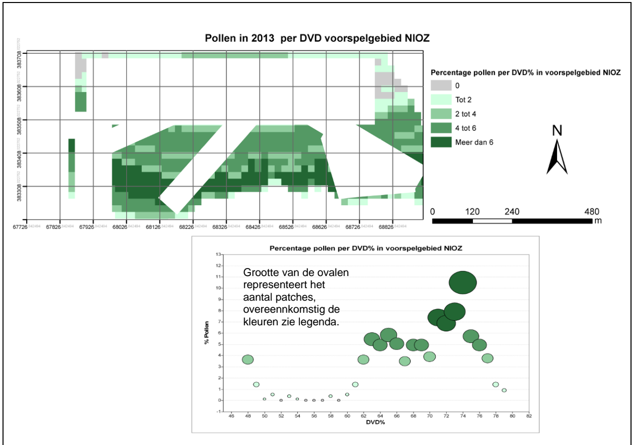
Figuur 14 Inschatting aantal en percentage pollen in 2013 in voorspelgebied NIOZ
