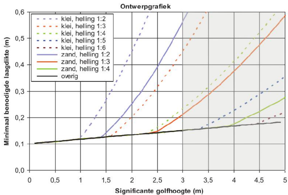
FIGUR 2-4 GRAFIEK VOOR HET ONTWERPEN VAN EEN BEKLEDING VAN WATERBOUWASFALTBETON OP GOLFKLAPPEN
