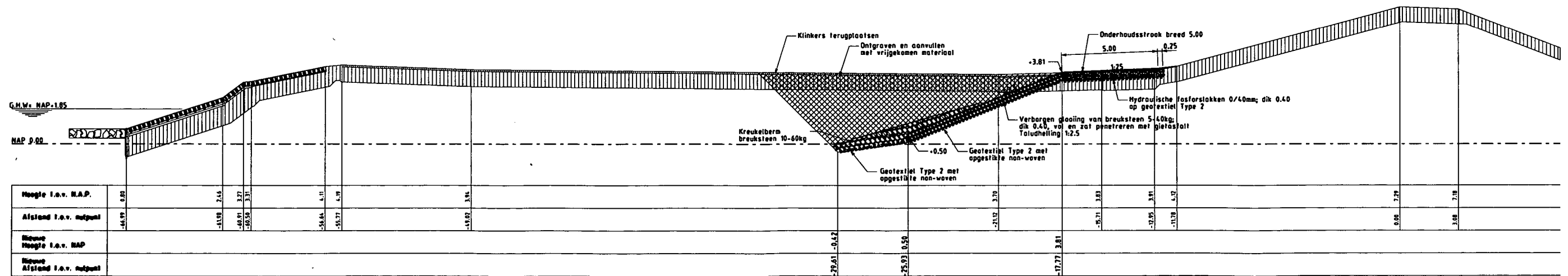
Dwarsprofiel 7 nieuw Van dp1270 tot dp1272-50m
