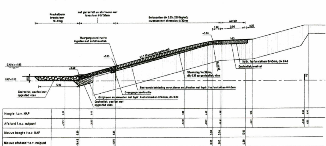
Dwarsprofiel 1: nieuw dp 1286
