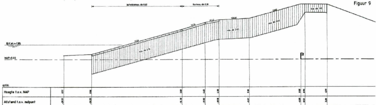
DWARSPROFIEL 1 bestand
