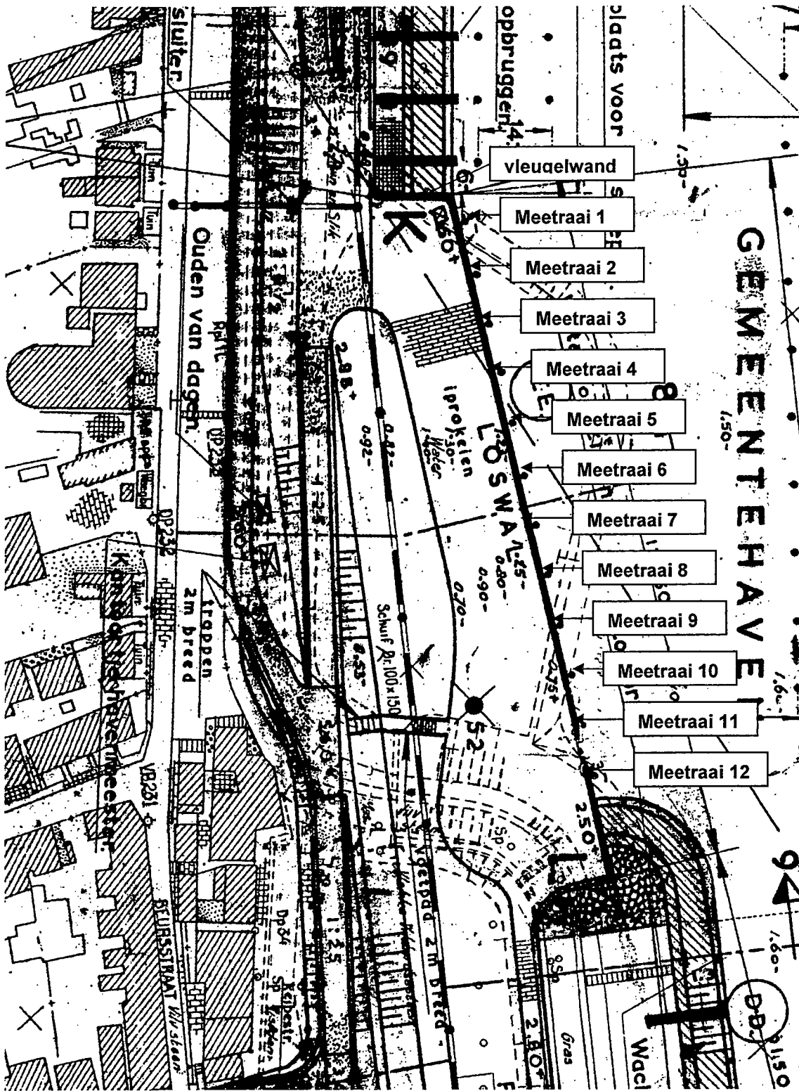
Overzicht meetraaien
