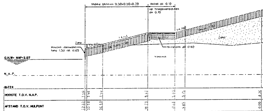
Dwarsprofiel 2 bestand
