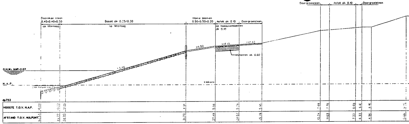
Dwarsprofiel 10 bestaand
