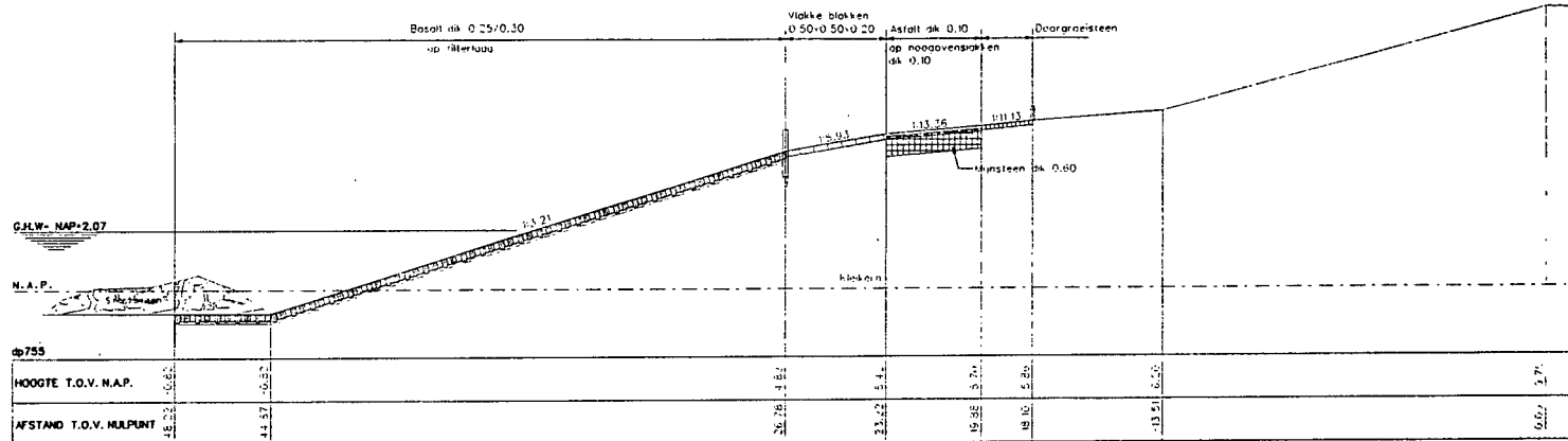
Dwarsprofiel 11 bestaand
