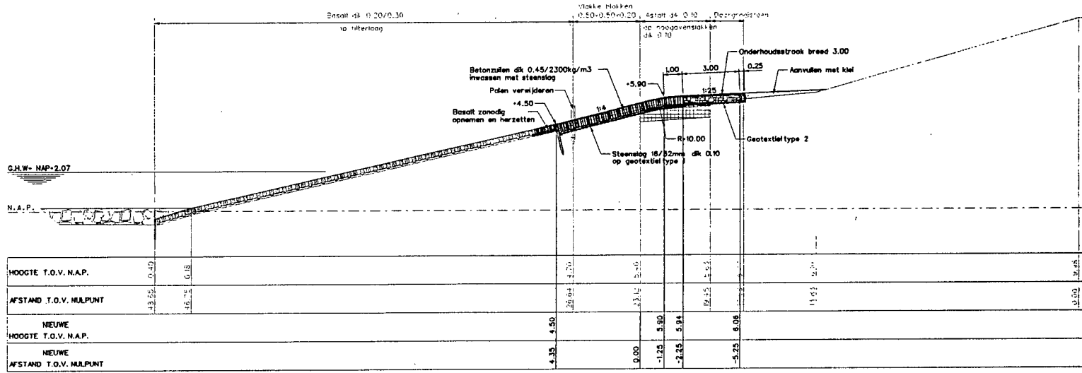
Dwarsprofiel 6 nieuw van d745+45m tot d747+35m
