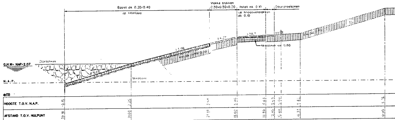
Dwarsprofiel 3 bestaand schaal 1:100
