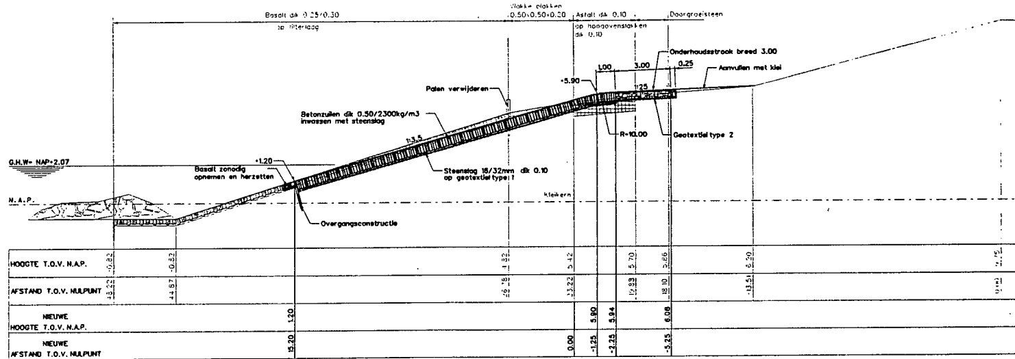
Dwarsprofiel 11 nieuw van 754 tot 756
