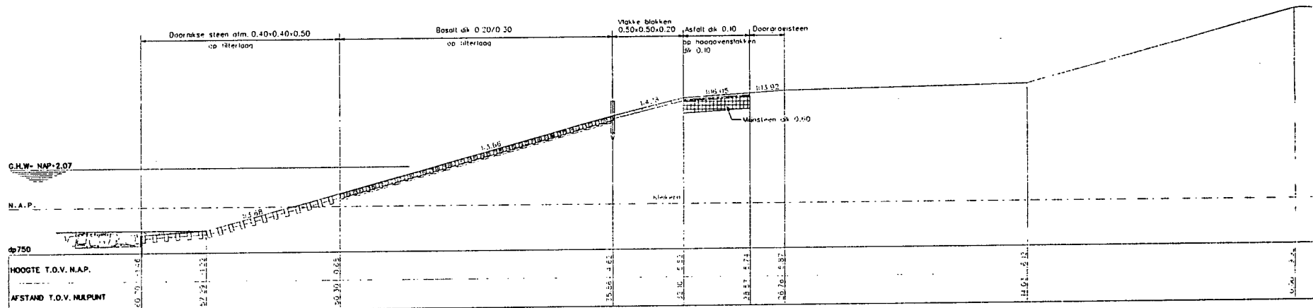
Dwarsprofiel 8 bestaand
