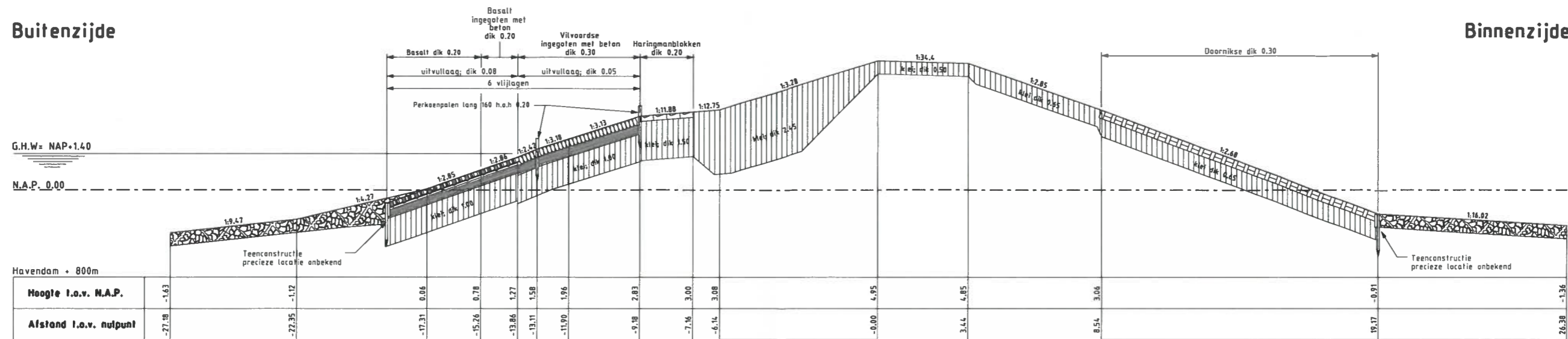
Dwarsprofiel 6 bestaand
