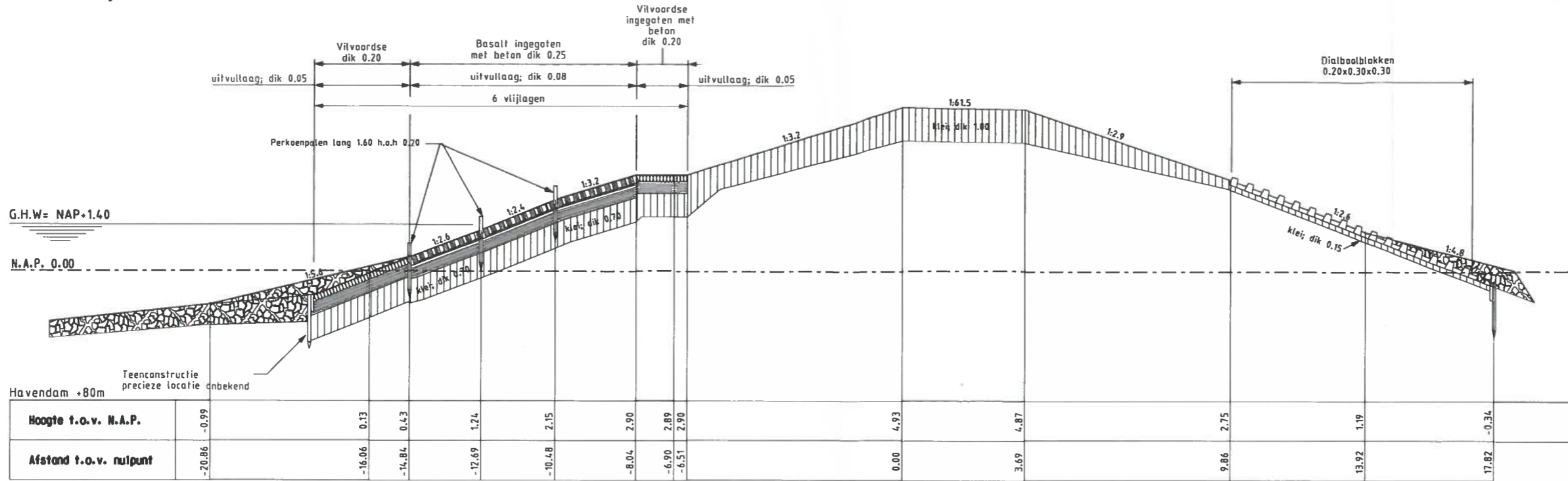
Dwarsprofiel 5 bestaand
