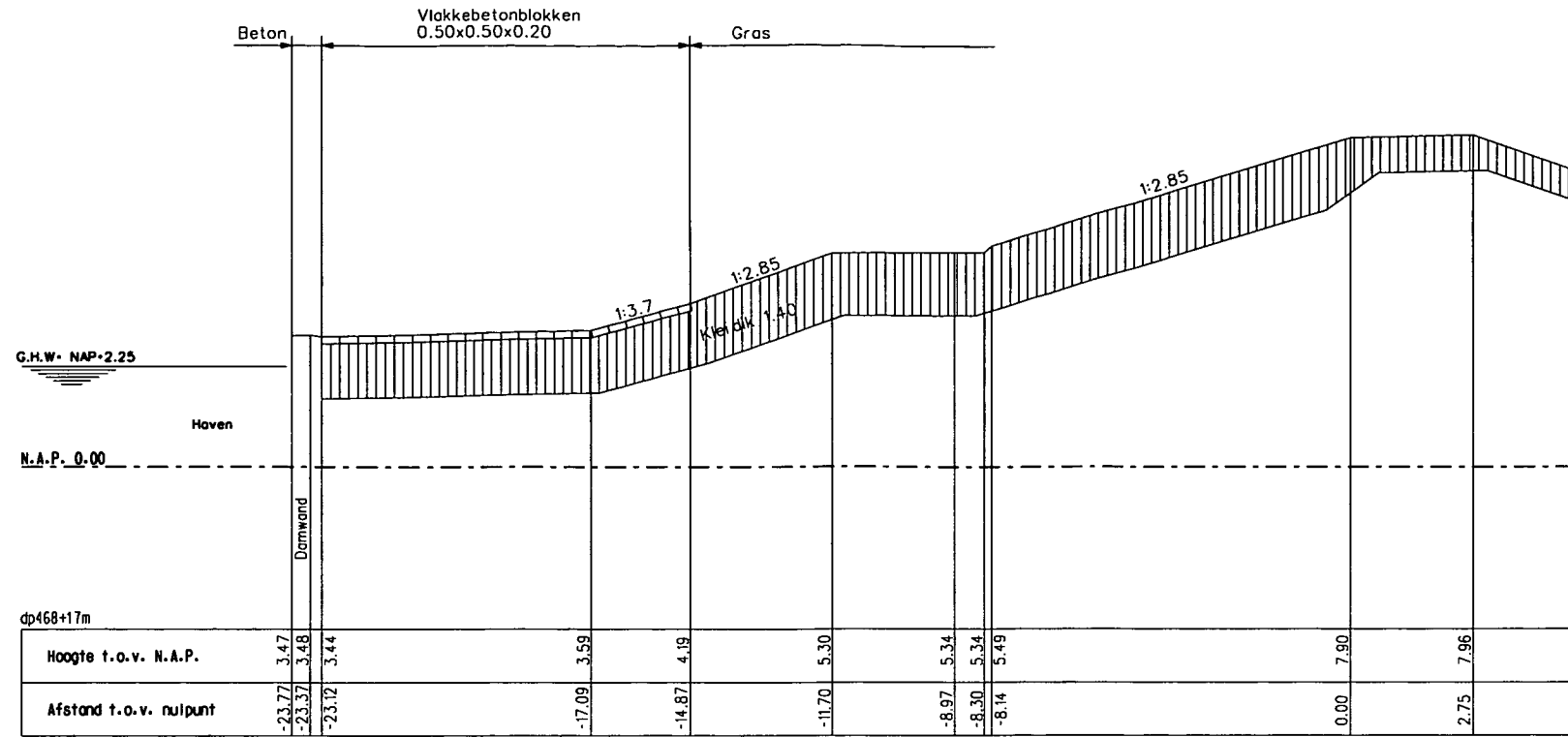
Dwarsprofiel 1 bestaand
