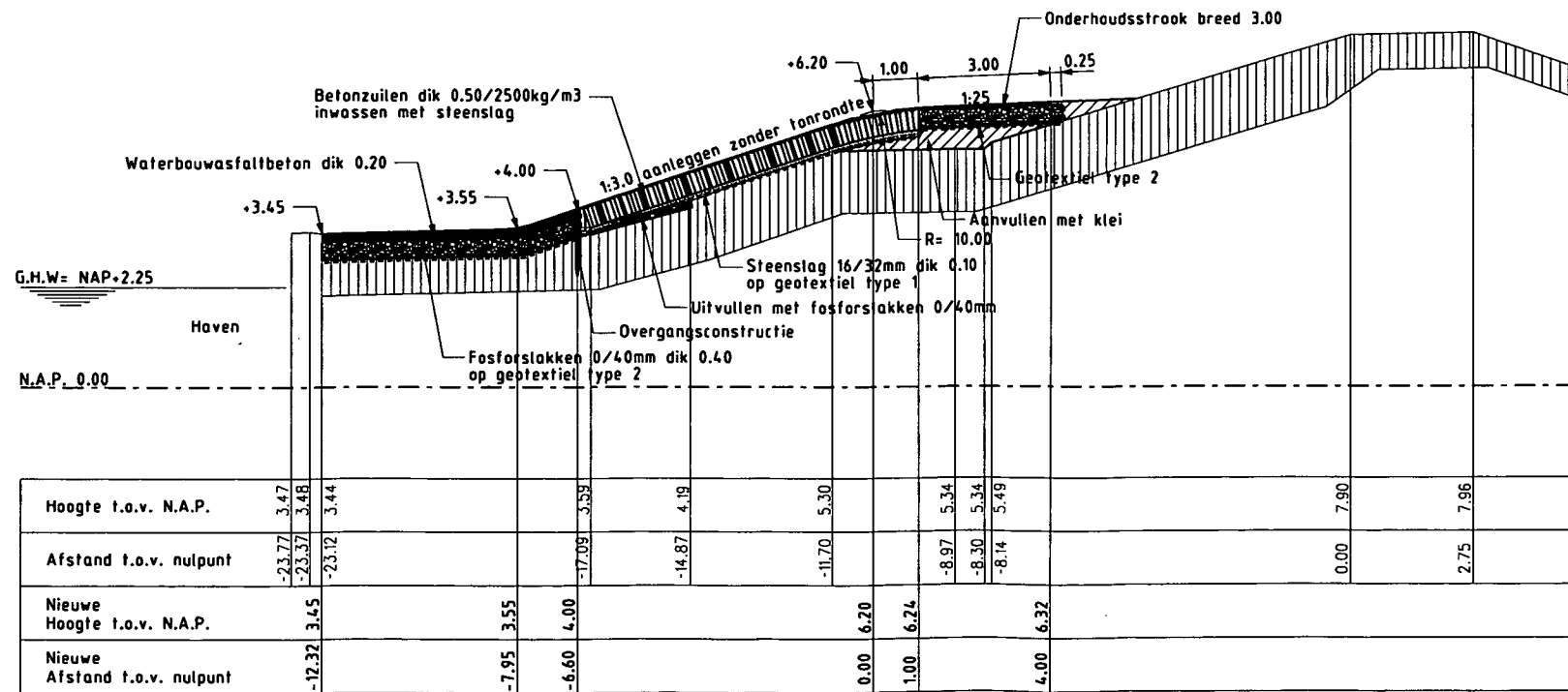
Dwarsprofiel 1 nieuw
