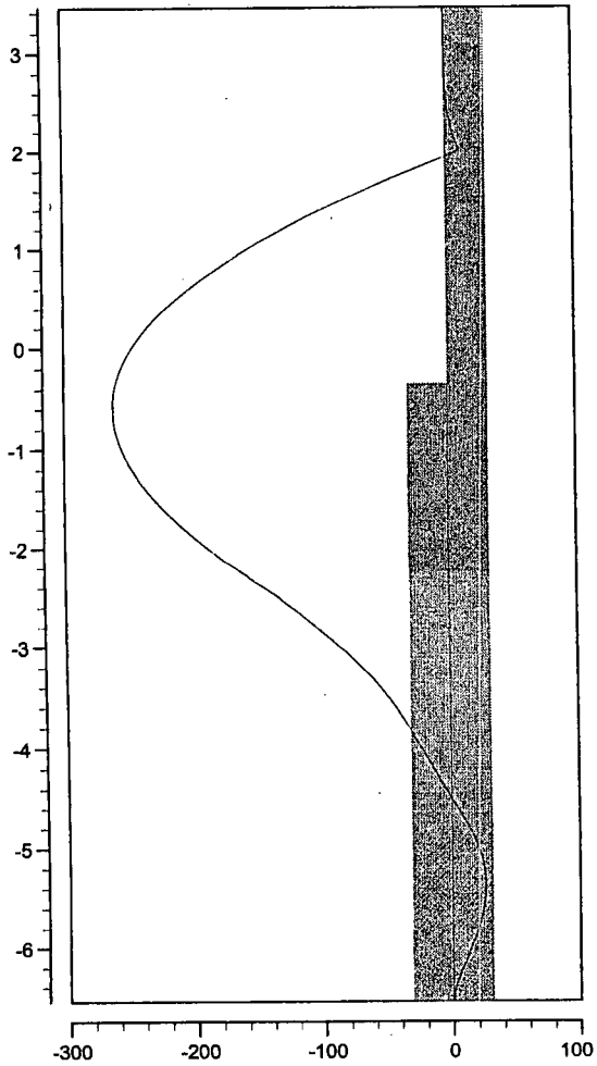
Buigende momenten [kNm/m 2 ]
