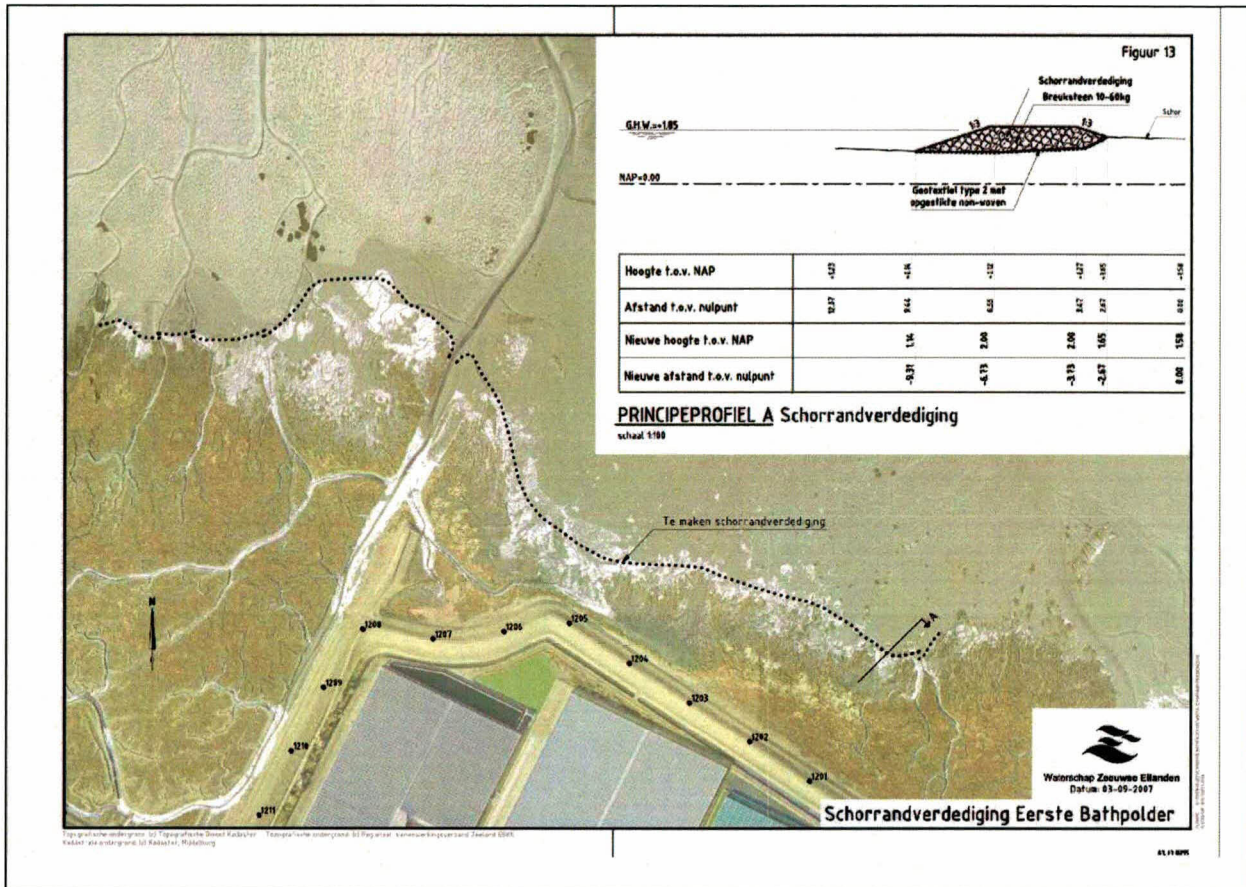
Figuur 2.4 Locatie en dwarsprofiel van de schorrandverdediging
