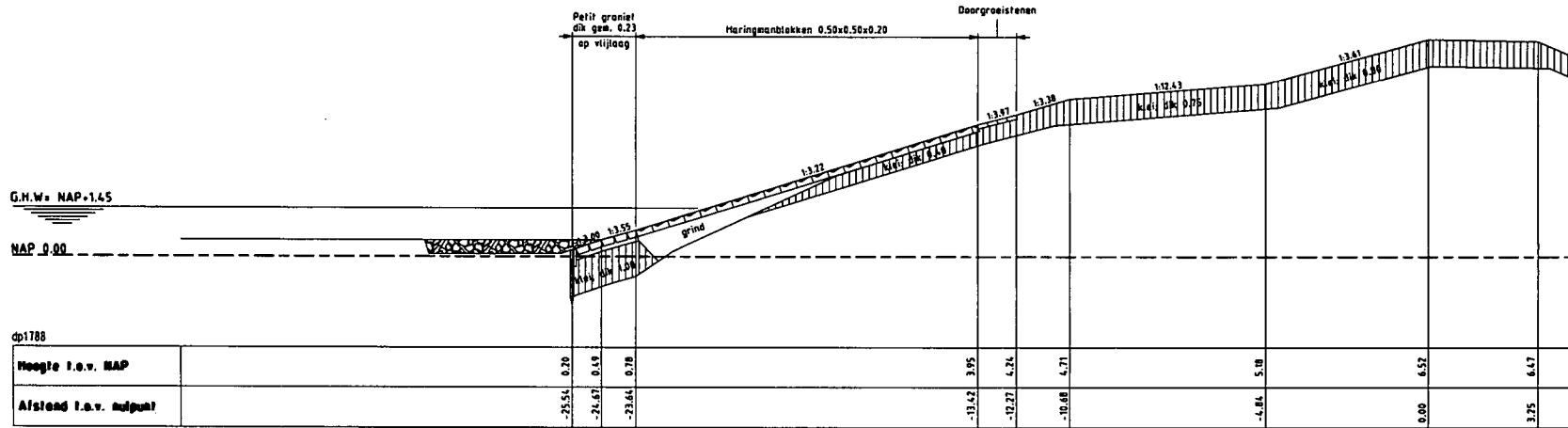
Dwarsprofiel 5 bestaand
