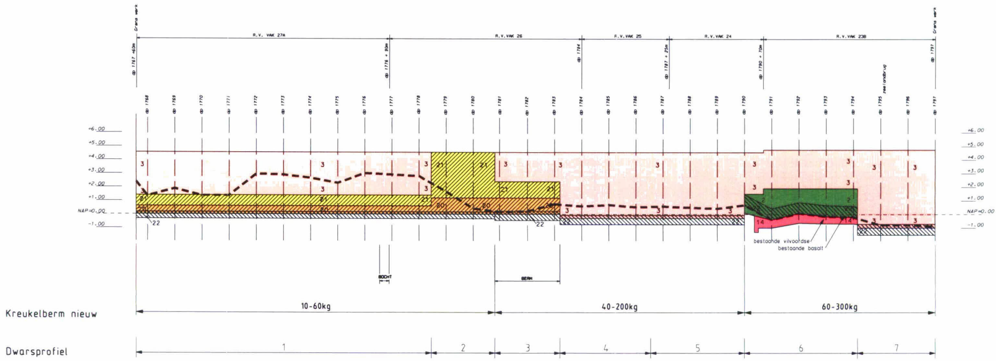
Figuur 6 Glooiingskaart Ontwerp alternatief 2
