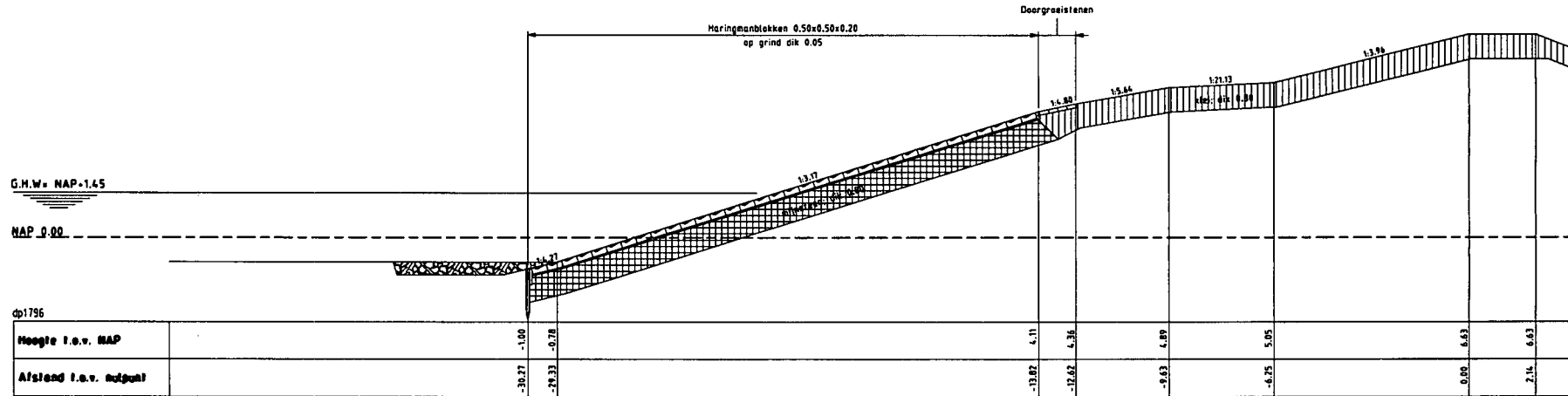
Dwarsprofiel 7 bestaand
