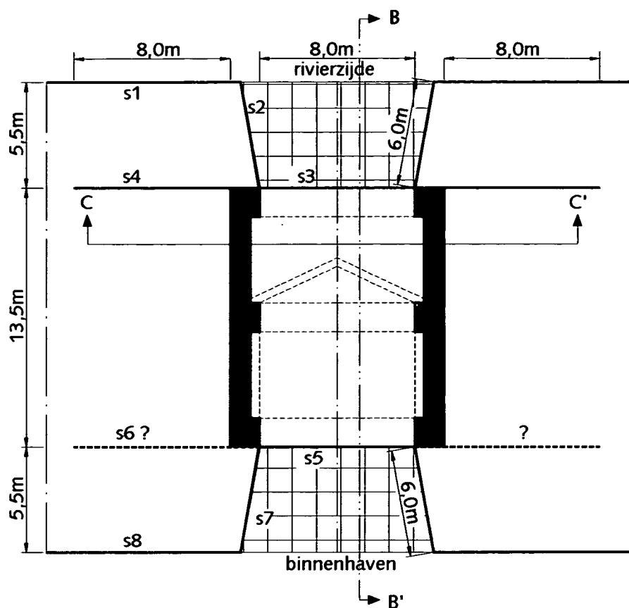
Figuur 7.3.3 Bovenanzicht (doorsnede A-A' in figuur 7.3.1)
