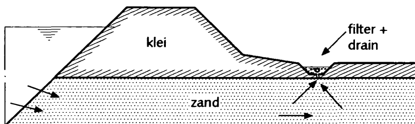
Figuur 3.4 Filterconstructie
