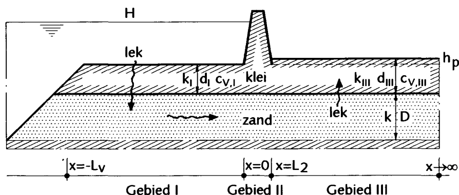
Figuur A.1.1: Ondergrondconfiguratie t.b.v. stijghoogteberekening t.b.v. opbarstcontrole
