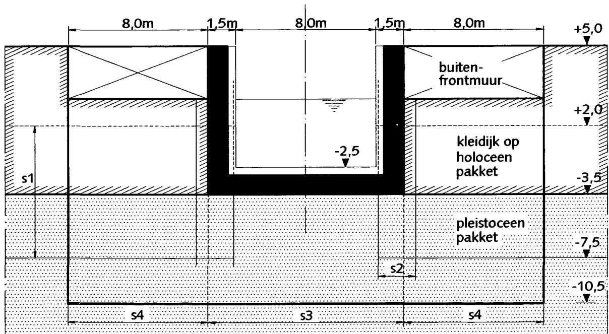
Figuur 7.3.1 Langsdoorsnede (doornede BB' in fig. 7.3.3)
