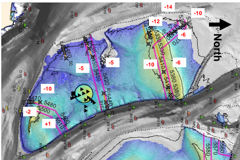
Figure 3-5 Erosion trends Galgeplaat RTK profiles [mm/y] (Santinelli 2011)
