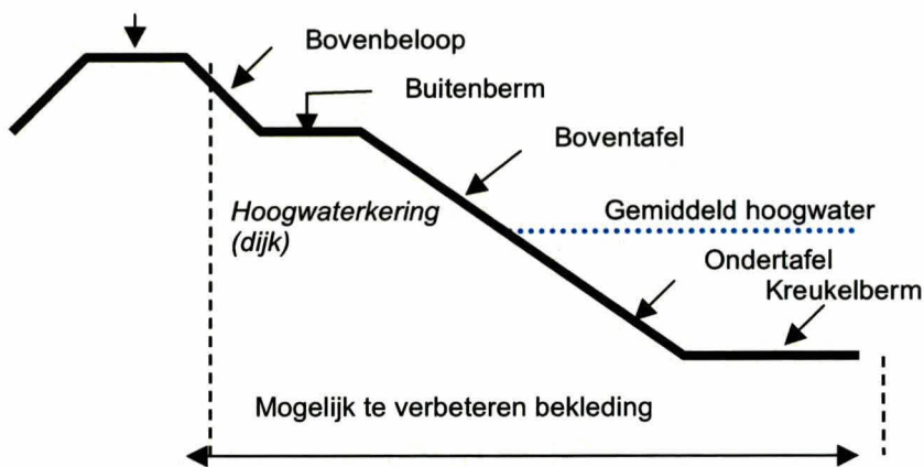
Doorsnede van een zeewering met namen van de diverse onderdelen.
