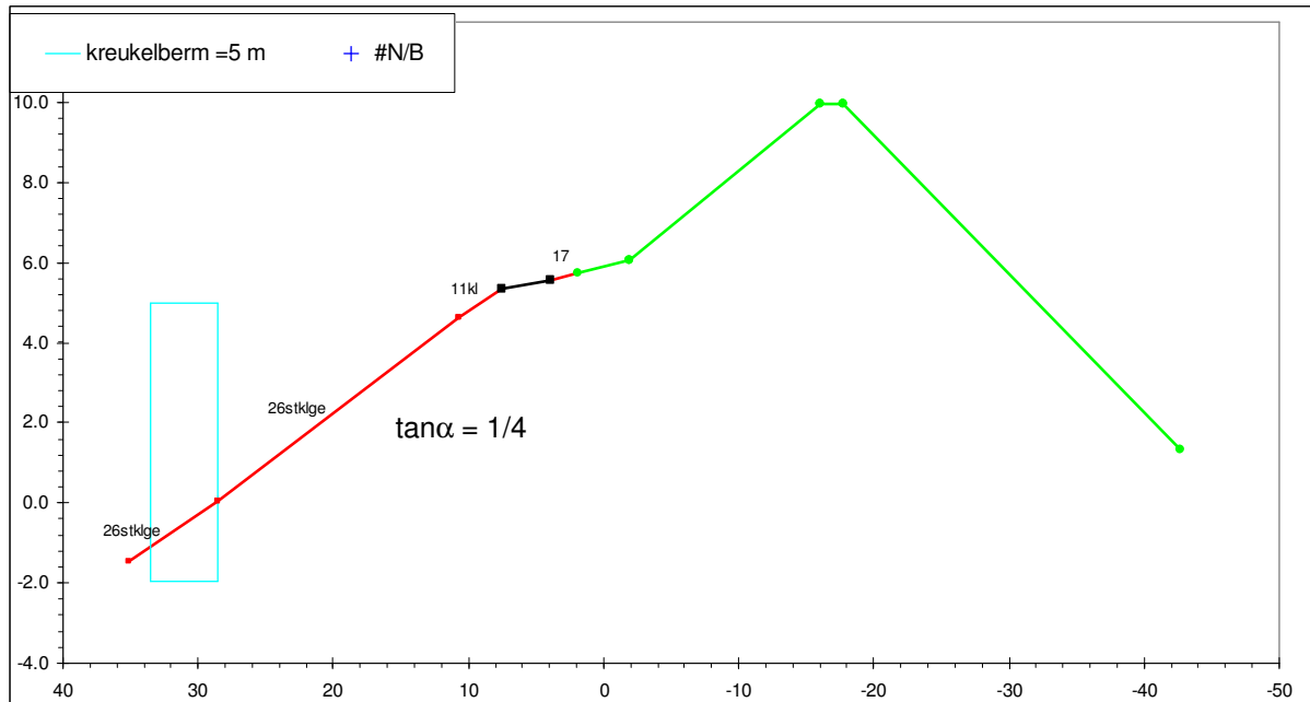
Profiel van case nr.4: Zuidwatering
