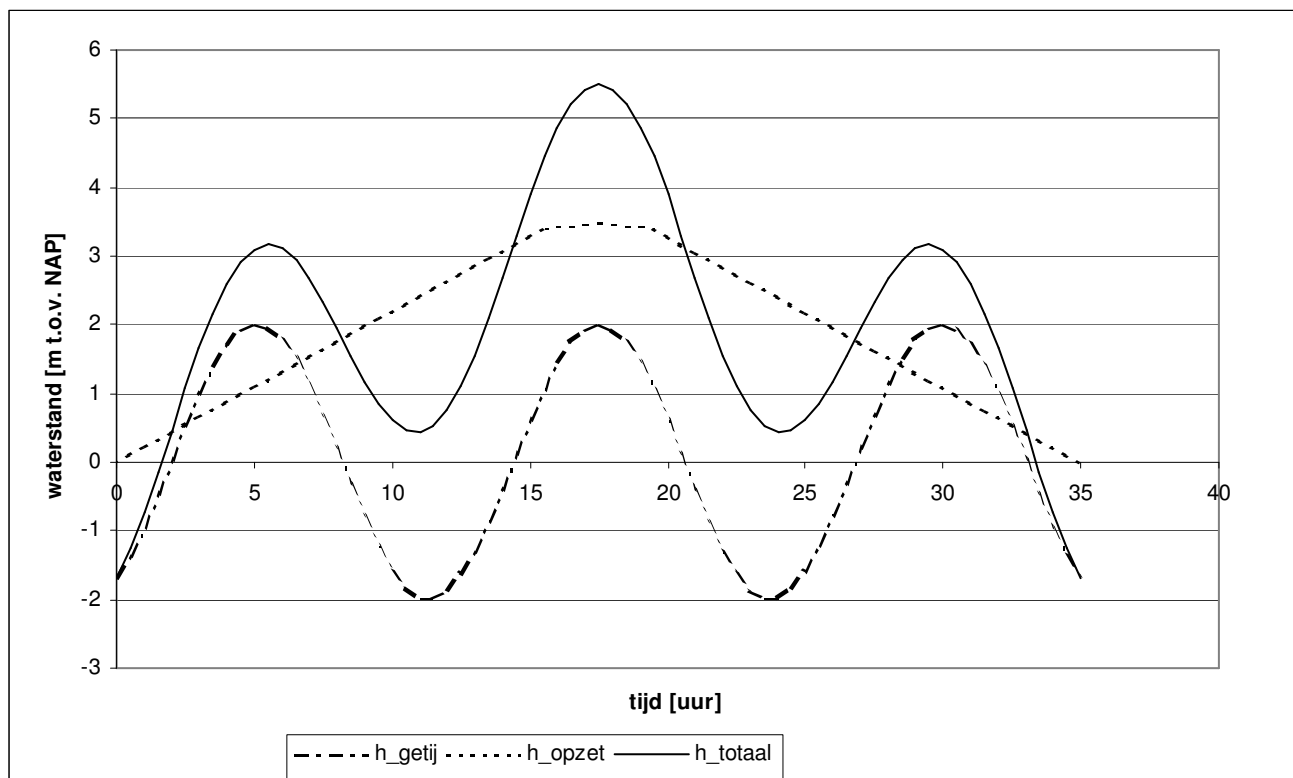
Figuur 3: Waterstandsverlooptlijn bij TP2006
