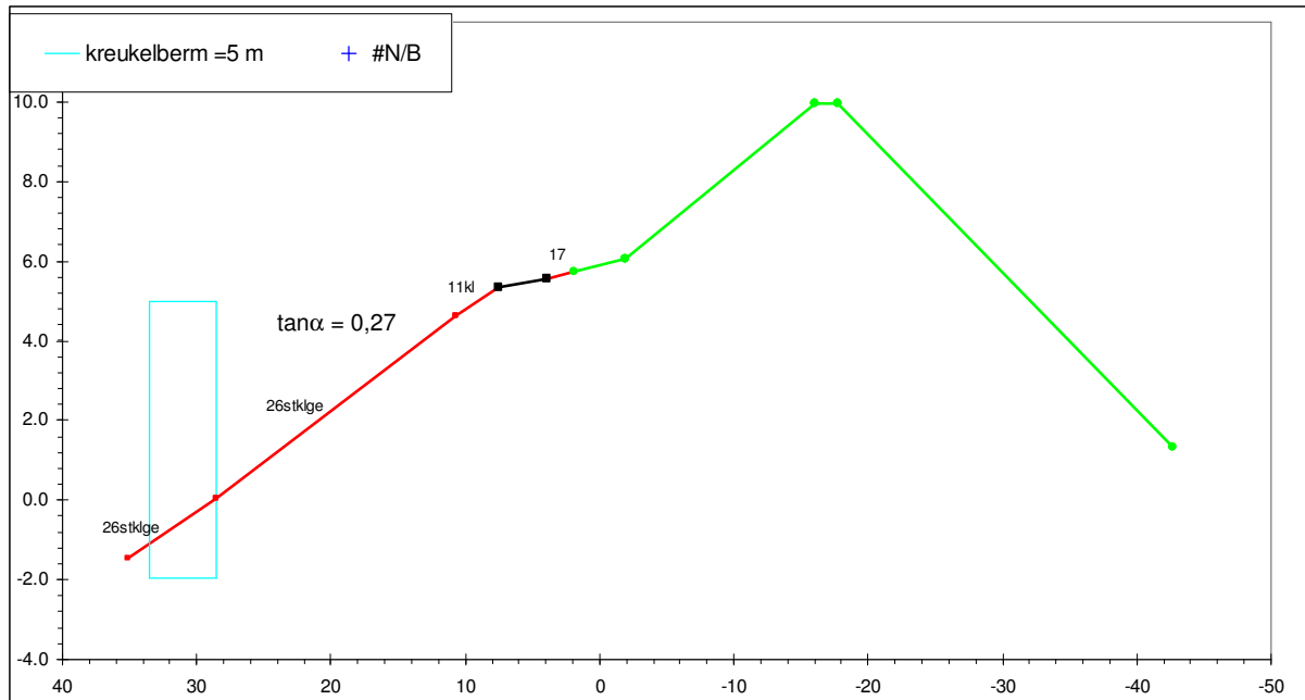
Figuur 2: Profielschets van profiel 4
