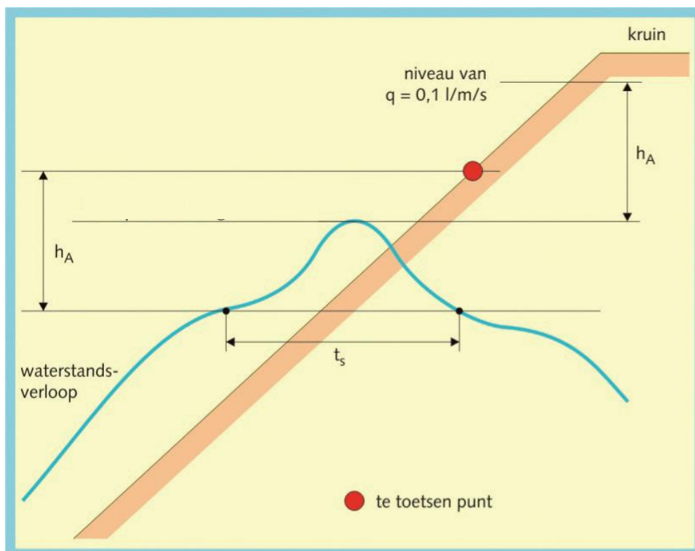
Figuur 4.11 Bepalen tijdsduur belasting t_s in de golfloopzone.
