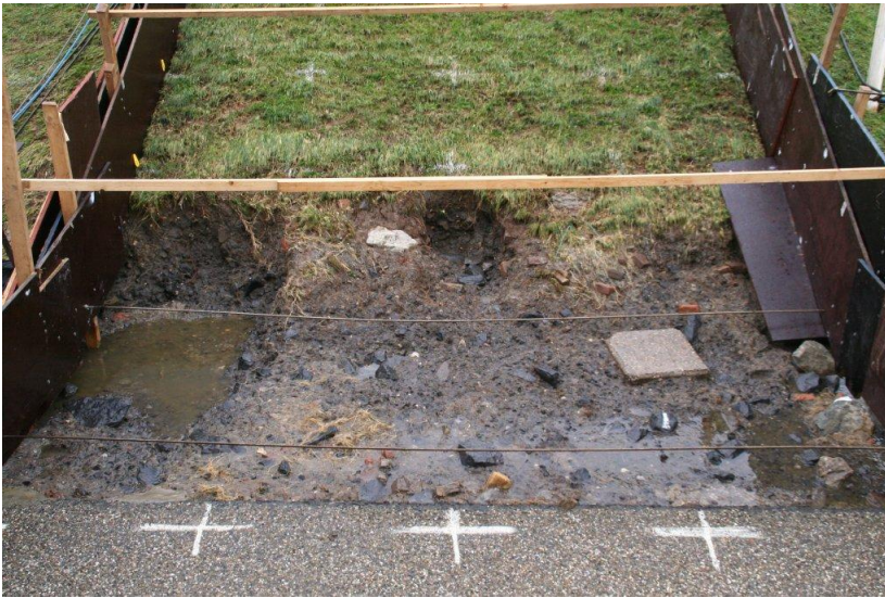
Figuur 5.9 Schade bij de overgang van buitenberm naar bovenbeloop van het buitentalud door golfoploop.
