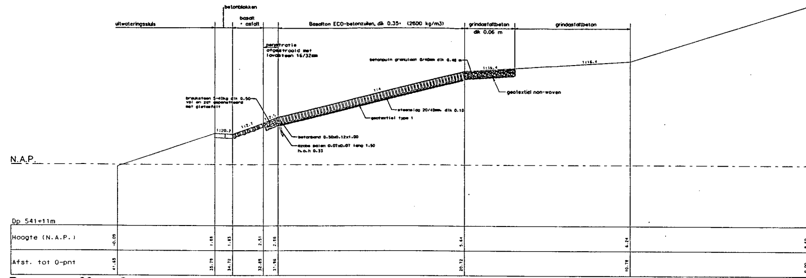
Dwarsprofiel 6 bestaand
