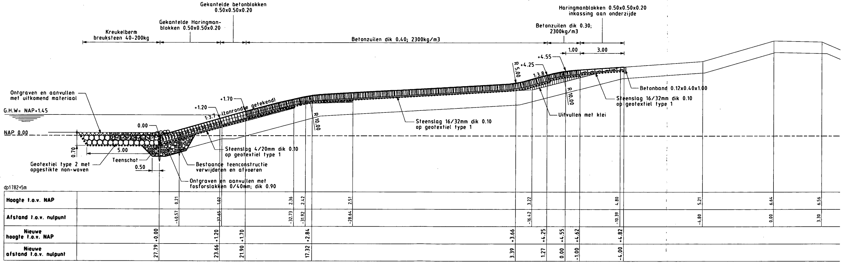
Dwarsprofiel 3 nieuw van dp1780.80m tot dp1783.20m schaal 1:100
