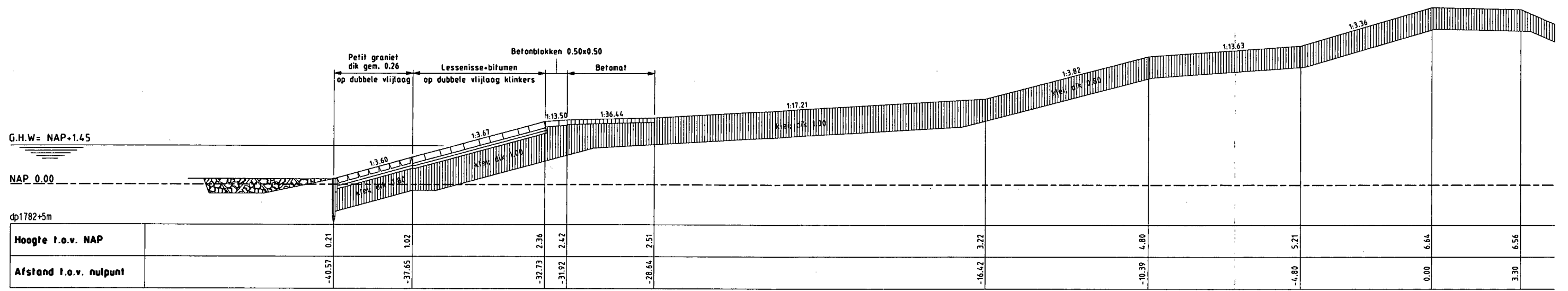
Dwarsprofiel 3 bestaand schaal 1:100
