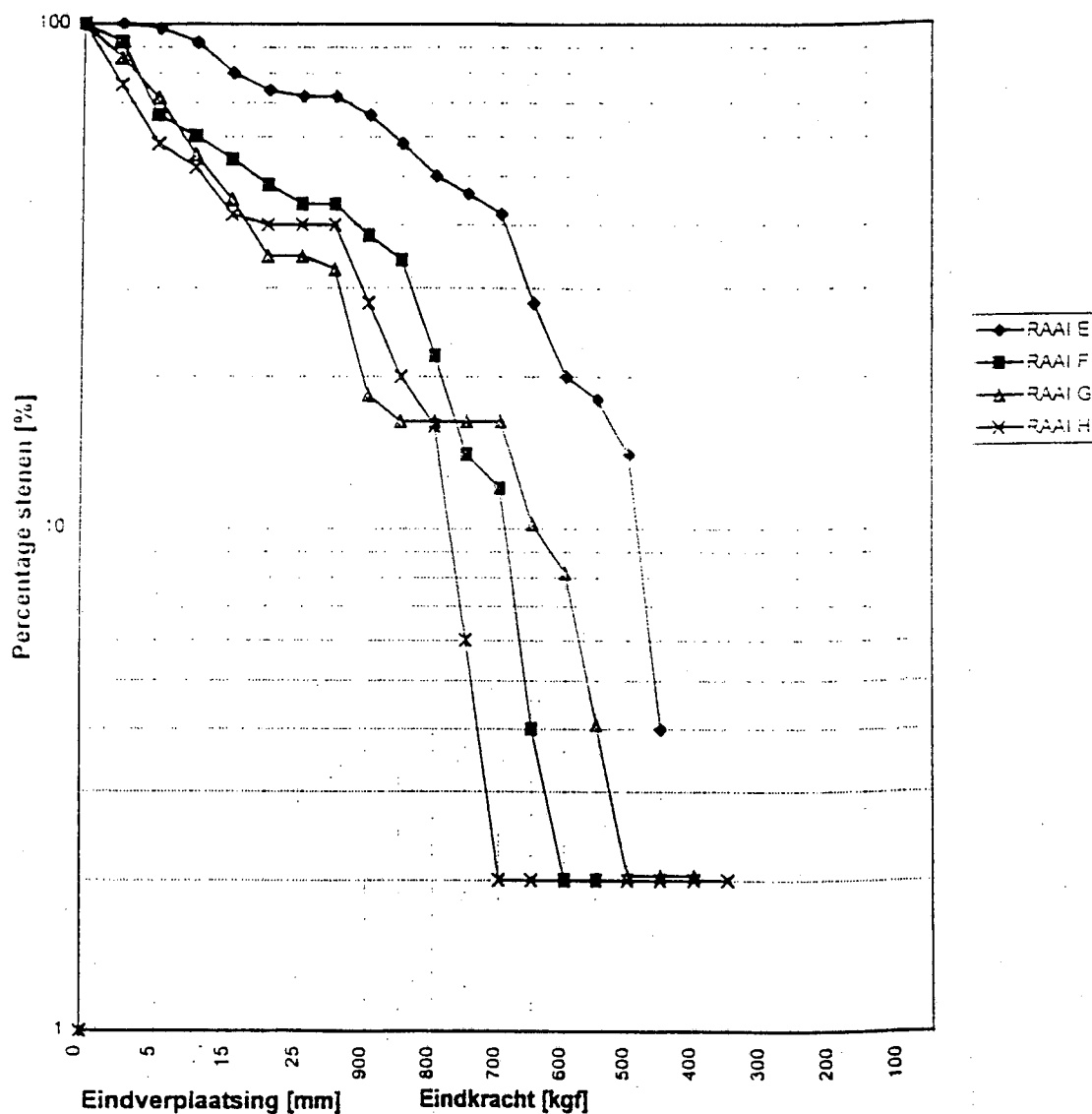
Grafiek 3: Percentage opgetreden krachten en verplaatsingen.
