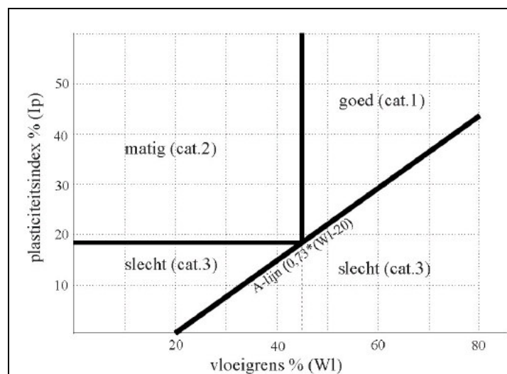
Figuur 2 Plasticiteitsdiagram voor bepaling erosiebestendigheid [Projectbureau Zeeweringen, 2008]
