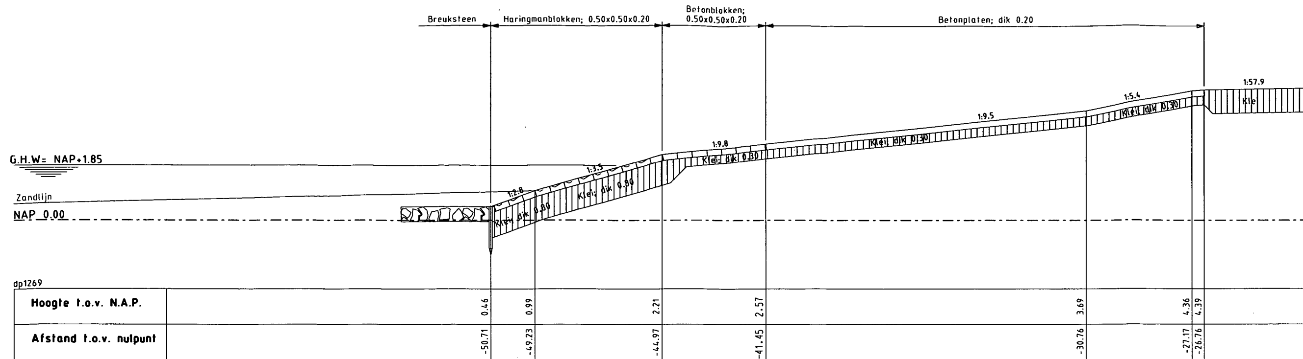
Dwarsprofiel 6 bestaand
