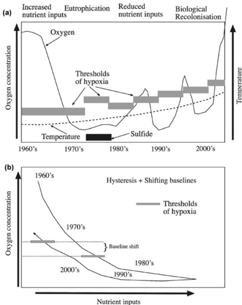
Figuur 3.3. Conceptuele diagram van de ontwikkeling van hypoxia drempelwaarden in relatie tot trends in vervuiling en temperatuur stijging. Dit leidt tot een verschuiving in de referentie waarde, naar hoger niveau (Steckbauer et al, 2011)
