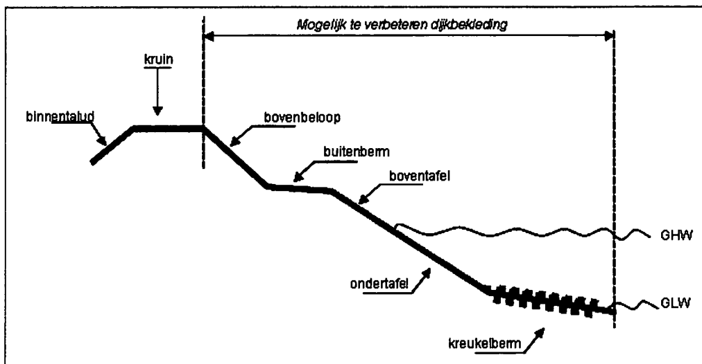
Figuur 2.1 Schematische weergave van het dijklichaam.
