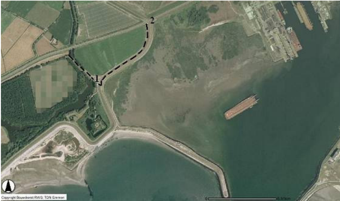
Figuur 2.4 Mogelijke tijdelijke opslagplaatsen en transportroutes bij de dijkverbetering
