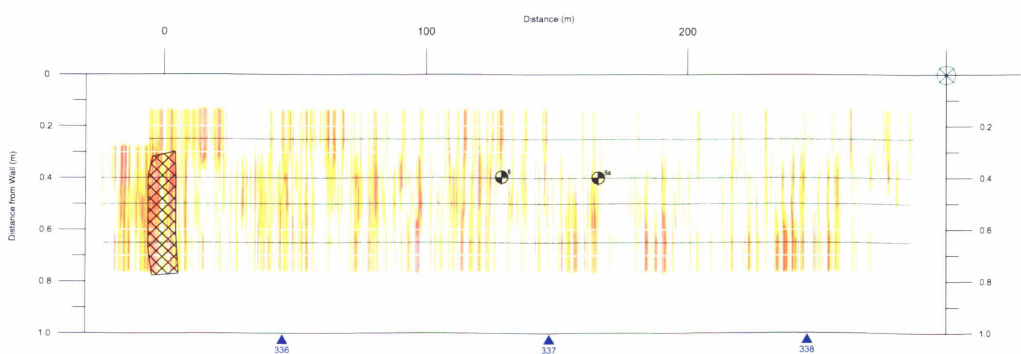
FIGURE 3: VIANE SECTION 2 DIJKPAAL 336 to DIJKPAAL 338
