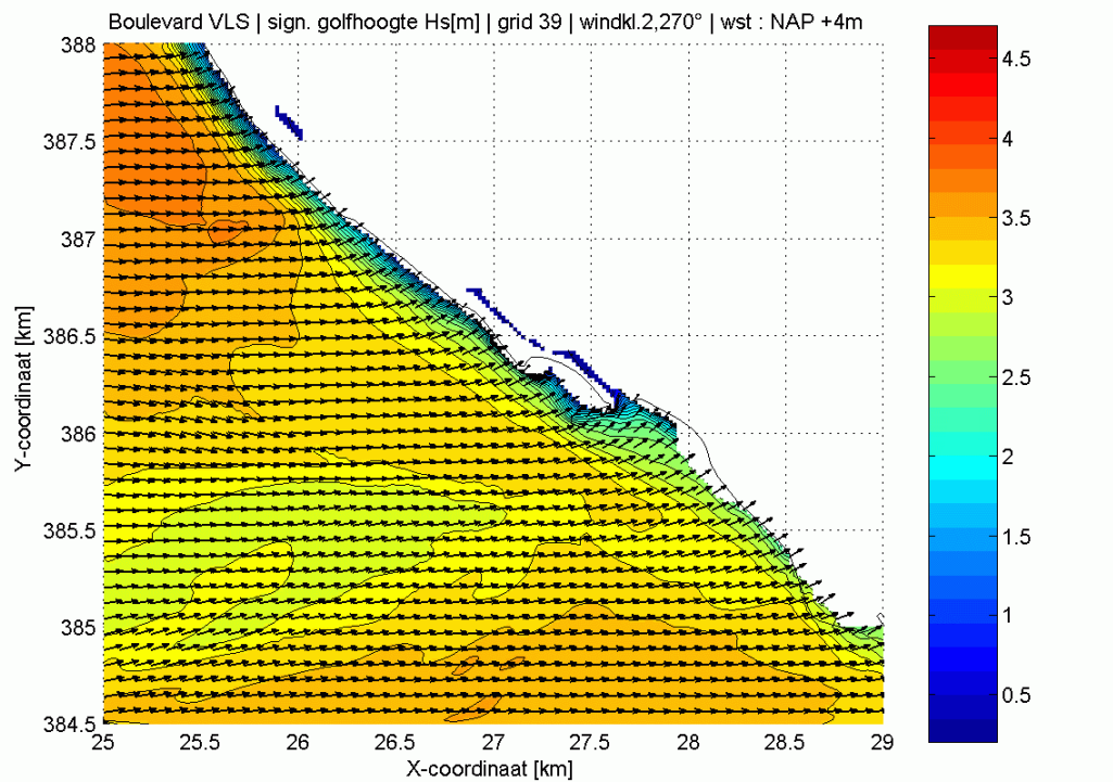
Figuur 2.1 en 2.2: Golfhoogte bij windrichting 270°, bij NAP4m en NAP+6m
