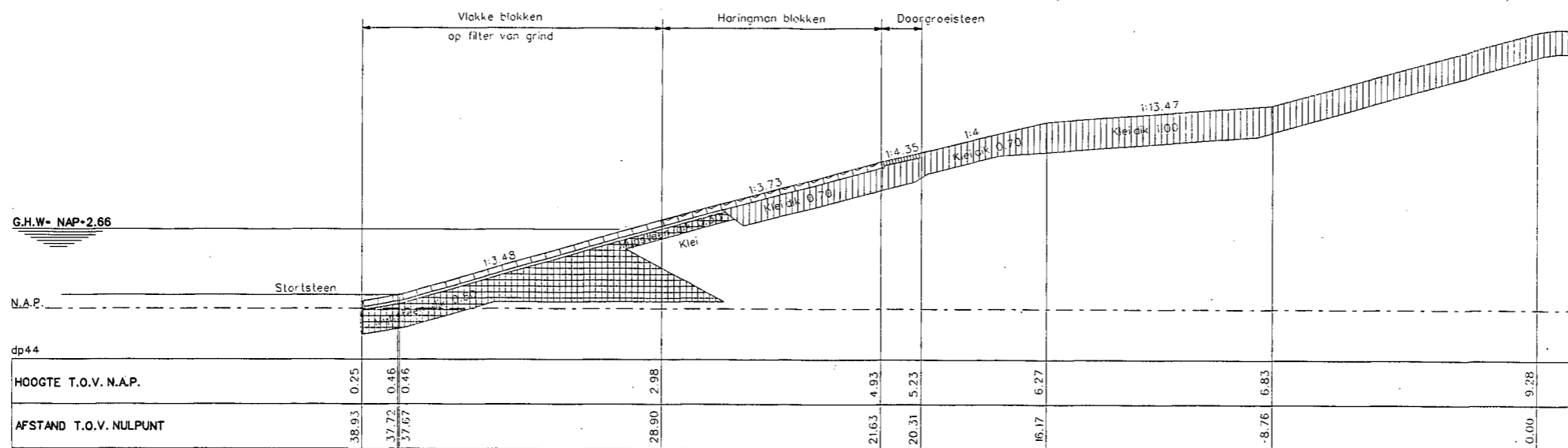
Dwarsprofiel 1 bestaand
