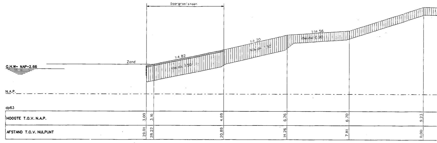
Dwarsprofiel 5 bestaand
