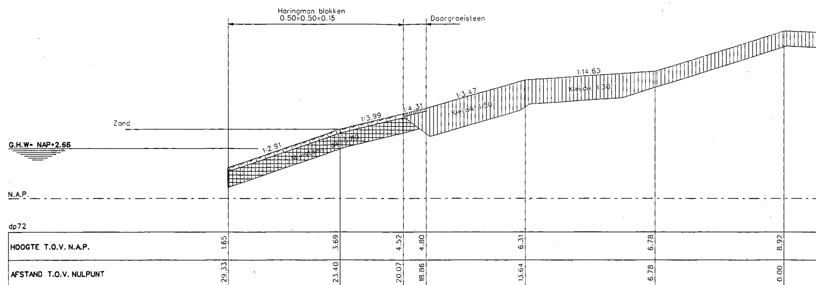
Dwarsprofiel 9 bestaand
