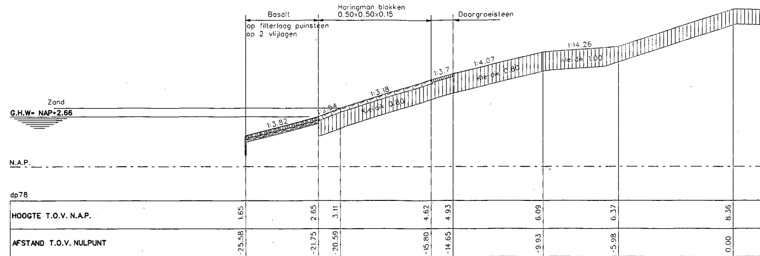
Dwarsprofiel 10 bestaand
