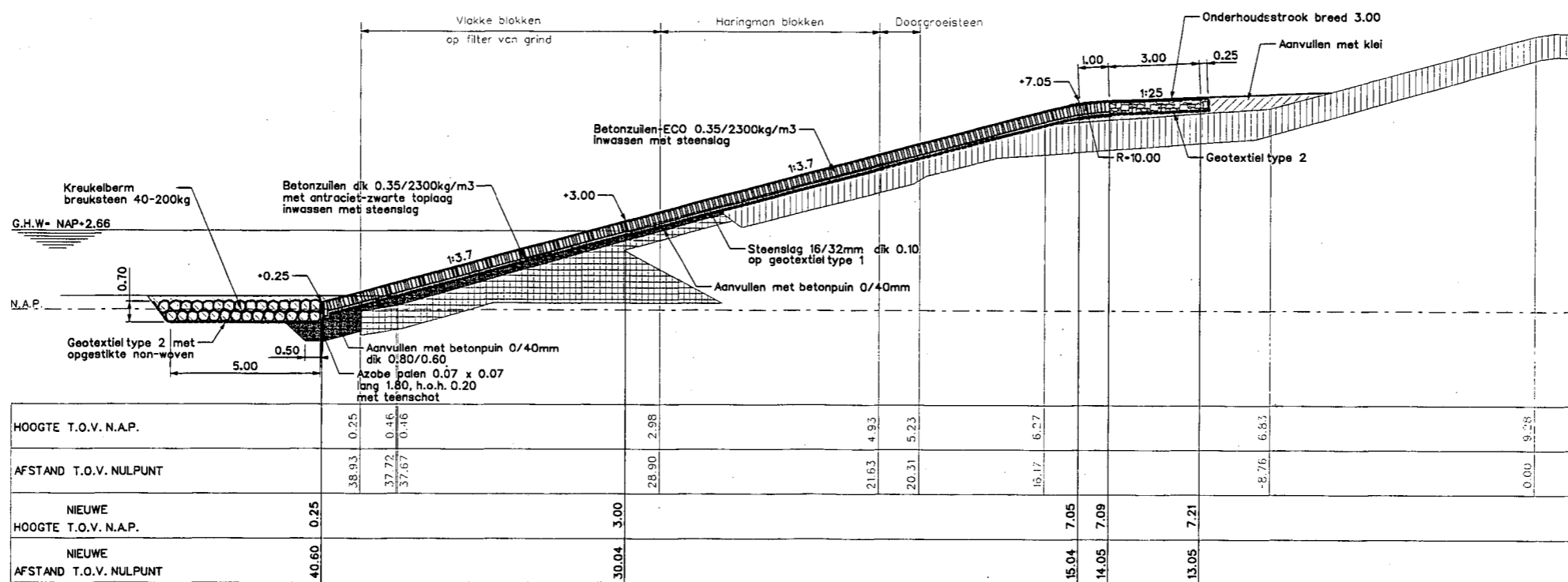
Dwarsprofiel 1 nieuw van dp43 tot dp44+75m
