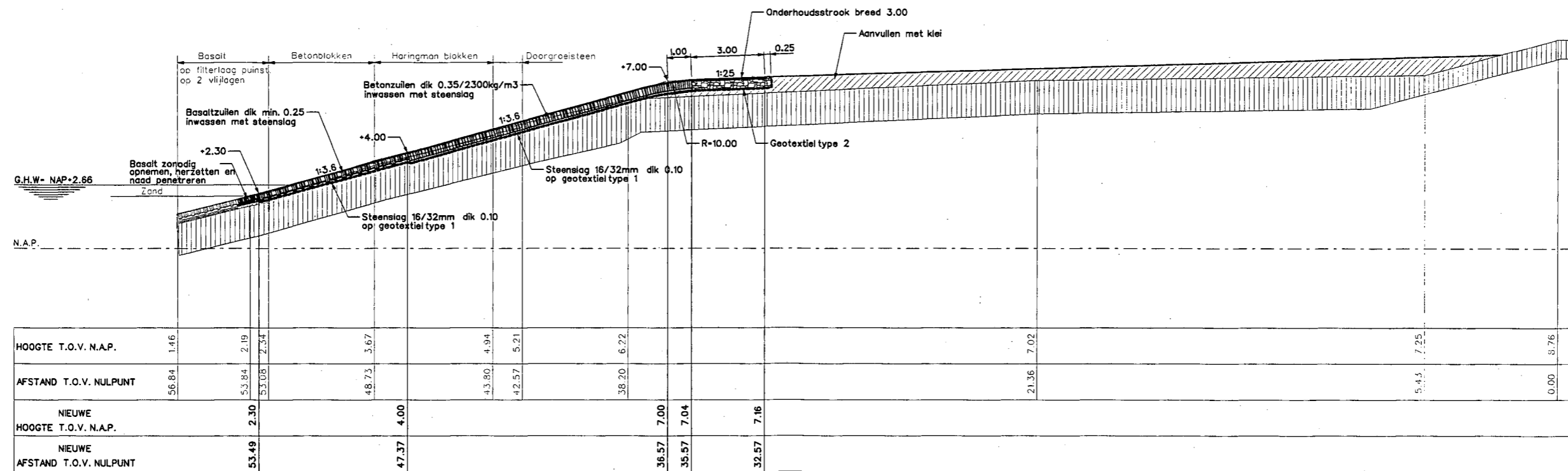
Dwarsprofiel 7 nieuw
