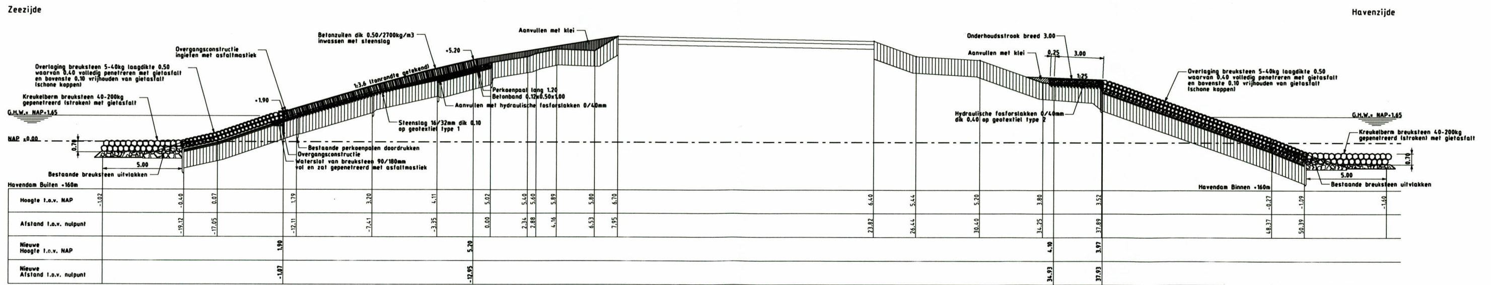
Dwarsprofiel 4 nieuw
