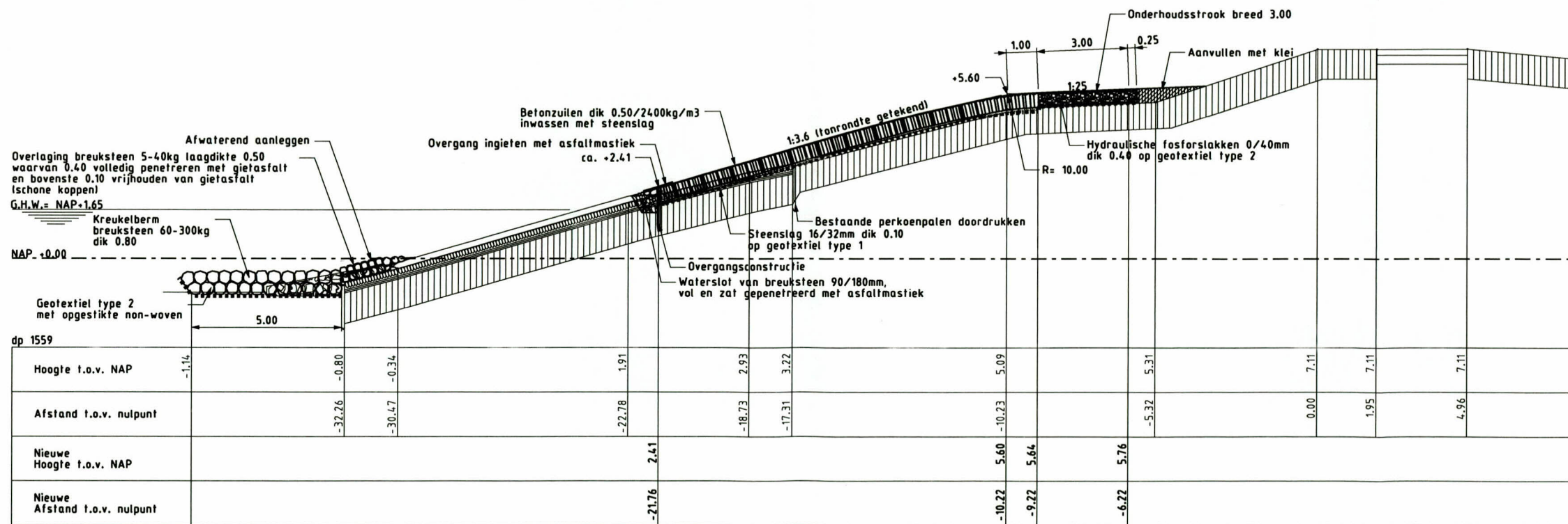
Dwarsprofiel 1 nieuw
