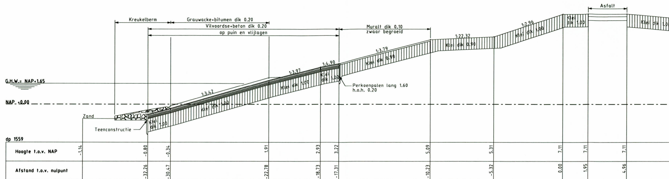
Dwarsprofiel 1 bestaand
