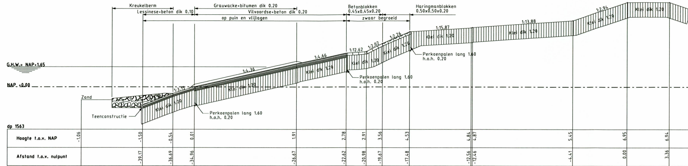
Dwarsprofiel 2 bestaand
