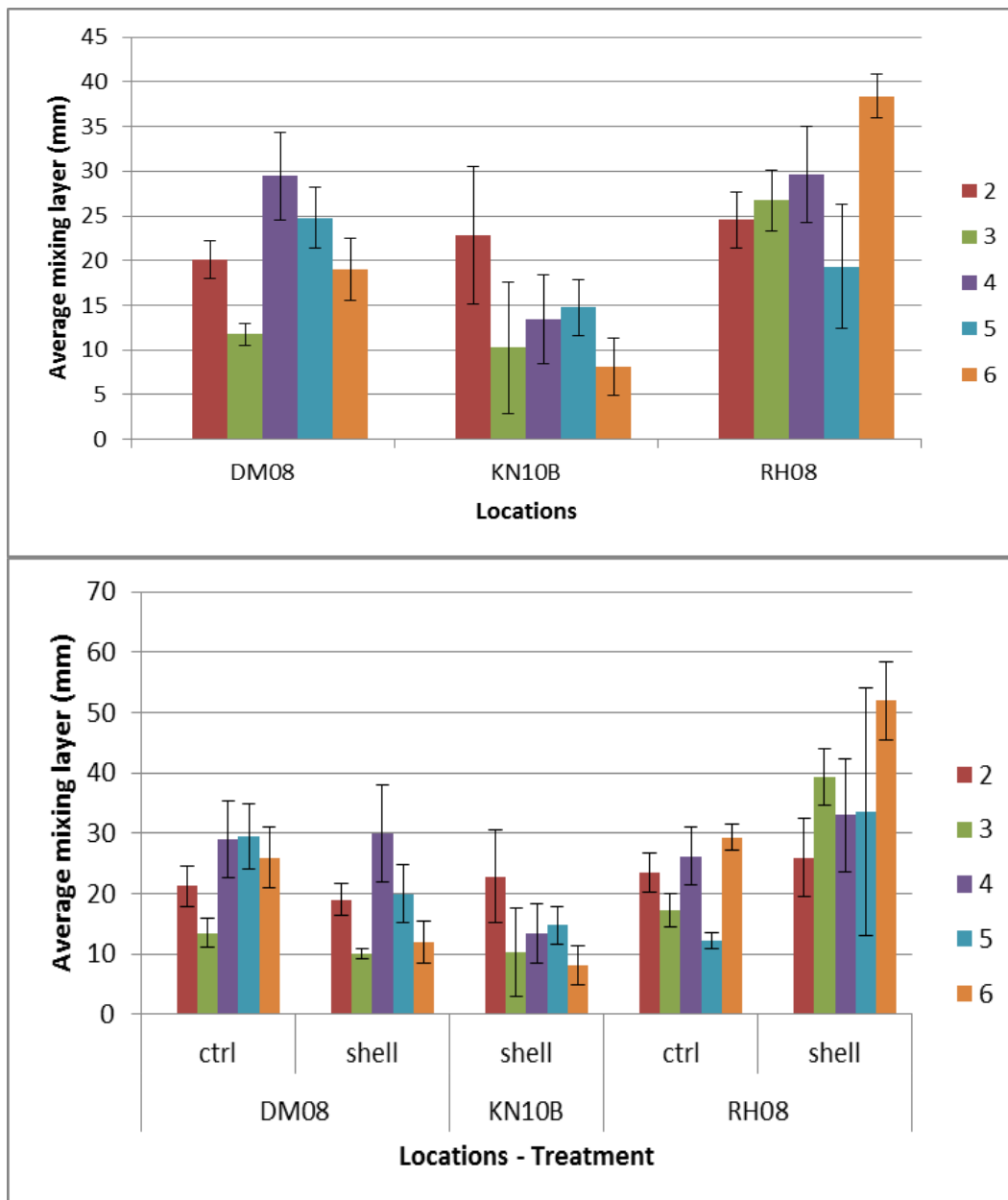
Figuur 43 Dikte van de mixinglaag over de gemeten intervallen per locatie (A, boven) en behandeling (B, onder) Errorbars geven standaardafwijking weer.
