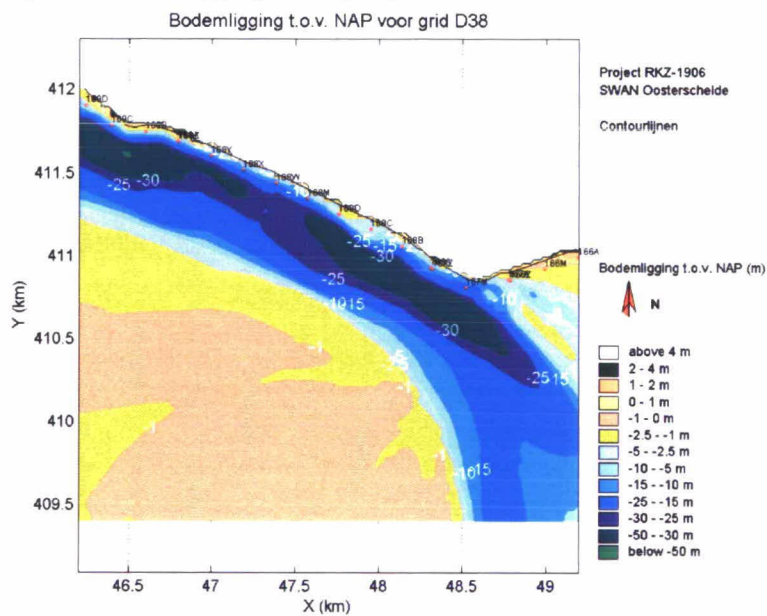
Figuur 4.1: Bodemligging rond dijktraject detailrooster D38
