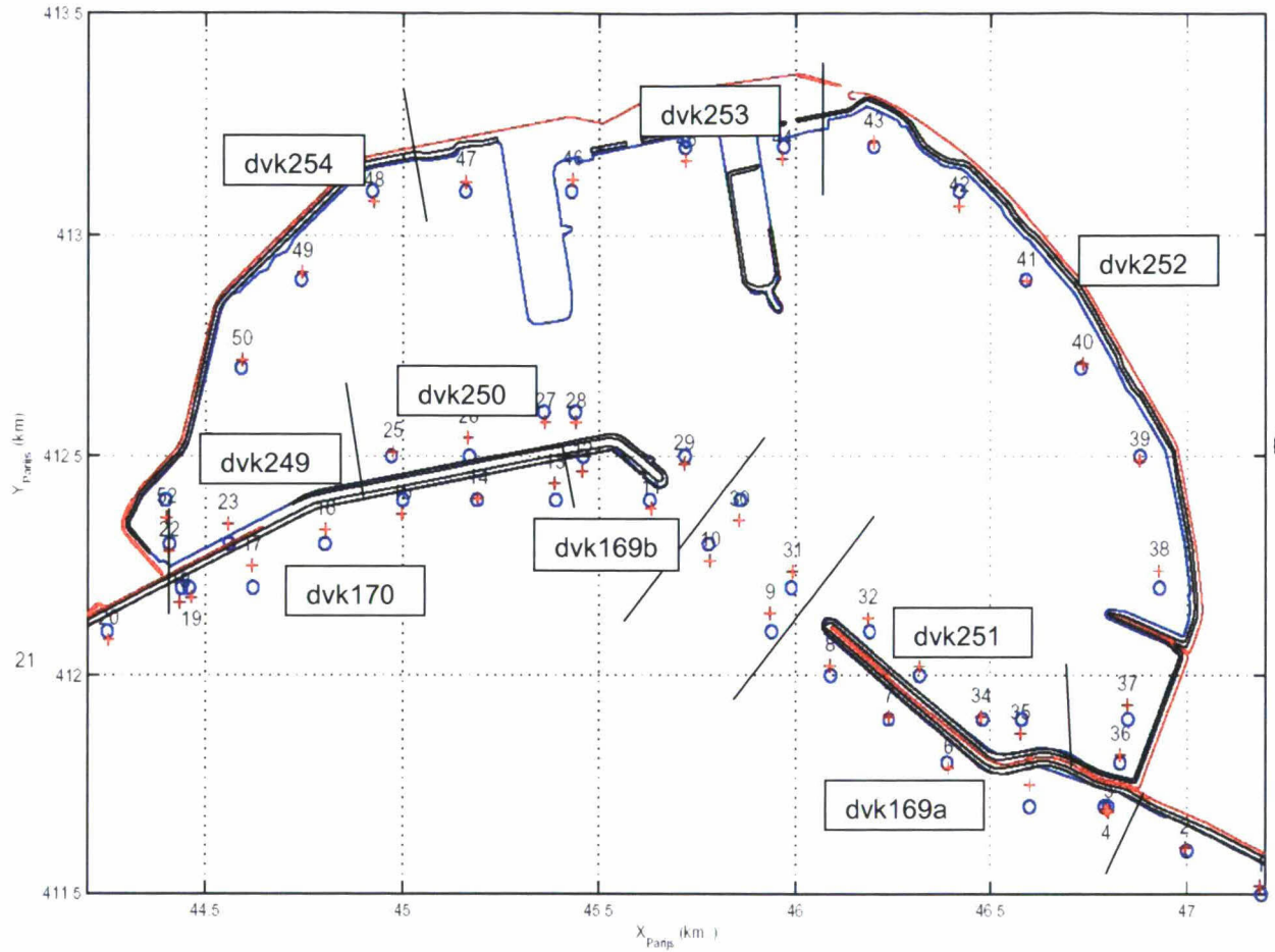
Figuur 1.4: Dijkvakindeling buitengebied en inlaagegebied Schelphoek en ligging SWAN-uitvoerpunten [ref 9]
