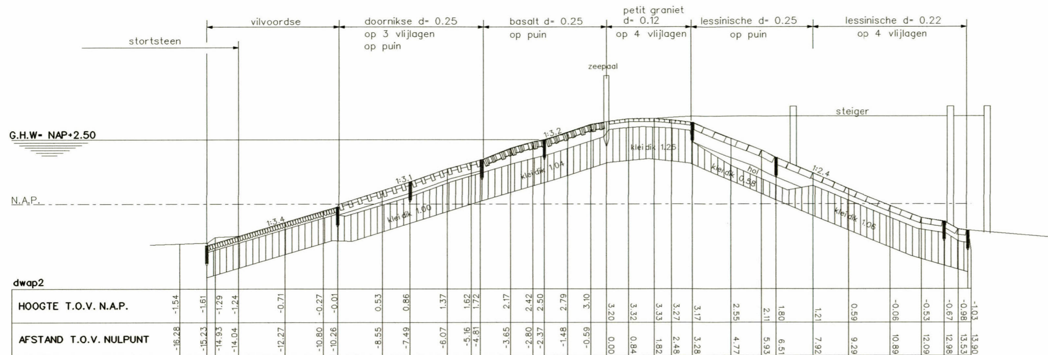
Dwarsprofiel 2 bestand
