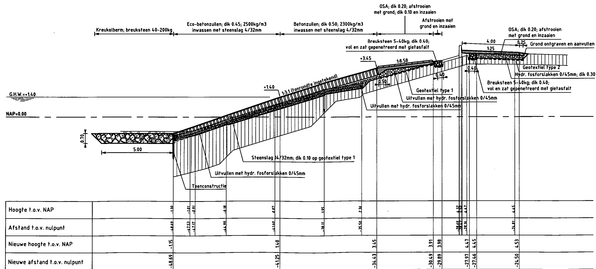
DWARSPROFIEL 1 nieuw van dp55 tot Havendam builen +0m
