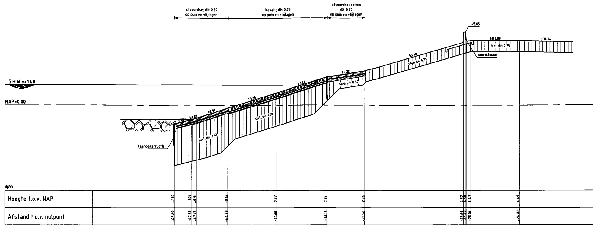
DWARSPROFIEL 1 bestand
