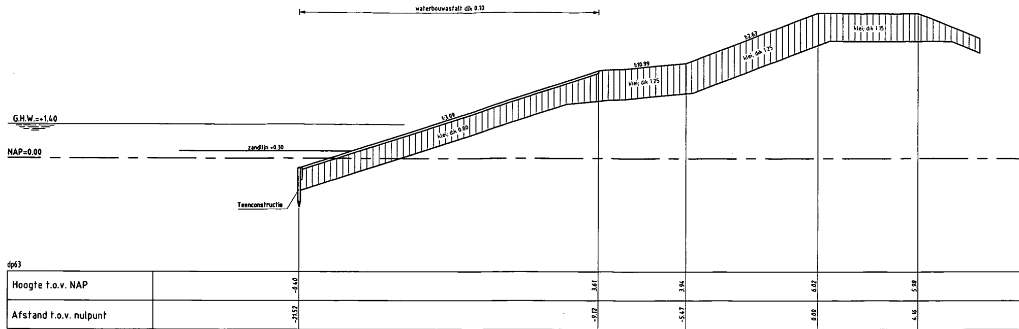
DWARSPROFIEL 6 bestand schaal 1:175
