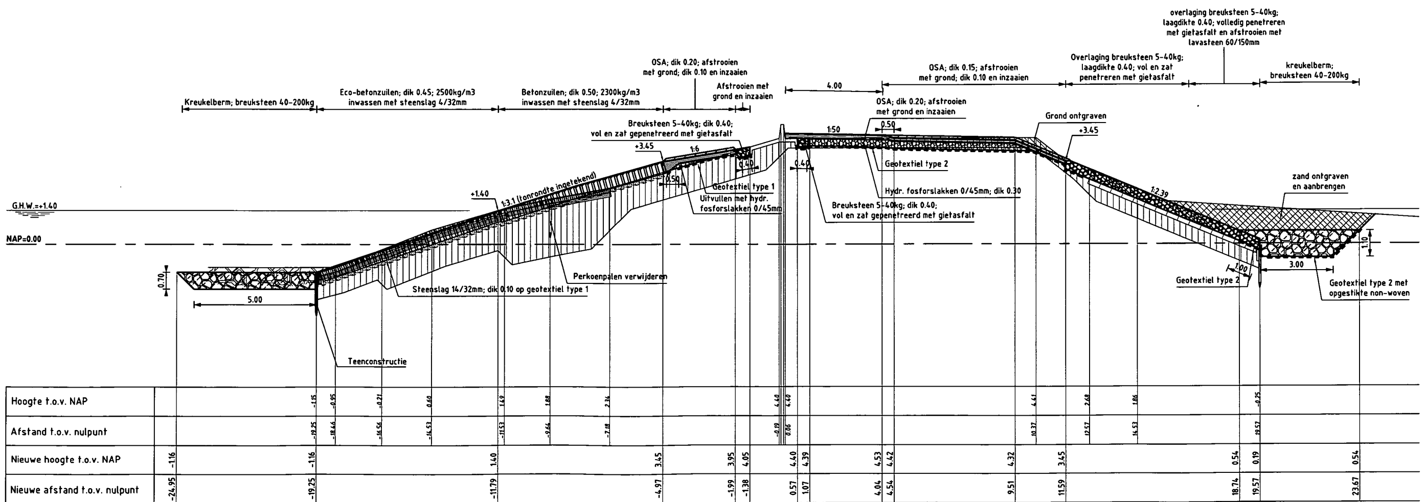
DWARSPROFIEL 2 nieuw van Havendam +0m tot Havendam +1000m (afstrooien overlaging van Havendam binnen +260m tot Havendam binnen +1000m) (van Havendam binnen +0m tot Havendam binnen +500m kreukelberm 10-60kg; dik 0.80 en bevind de teen zich op N.A.P. +0.40m) (van Havendam buiten +500m tot Havendam buiten +1000m komt teenconstructie op N.A.P. -1.50m)
