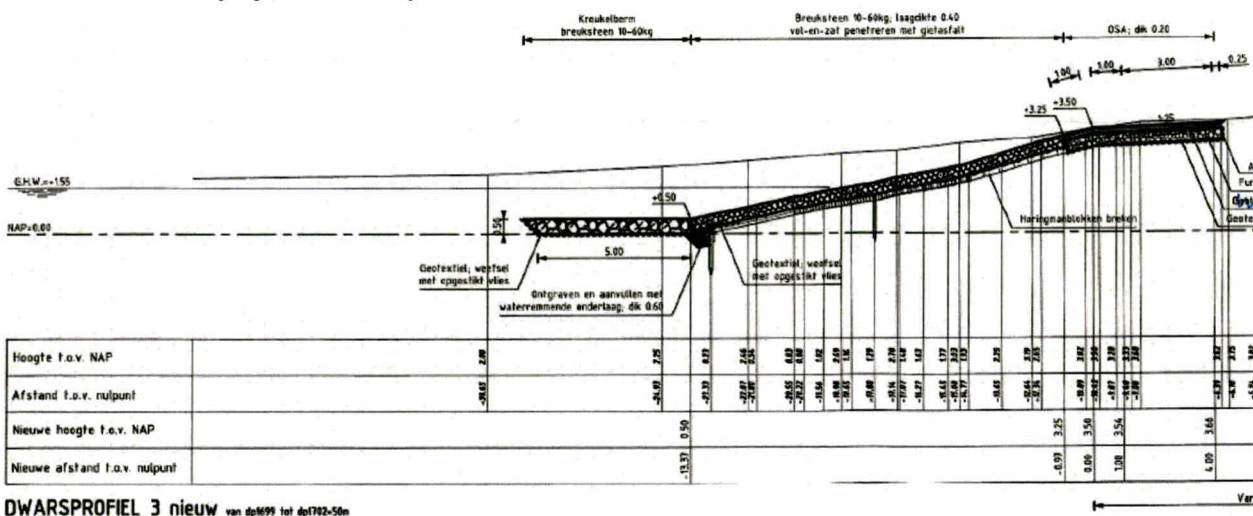
Dwarsprofiel 3: nieuw dp 1701
