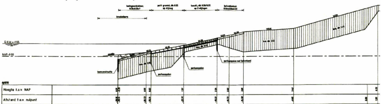
DWARSPROFIEL 2 bestaand
