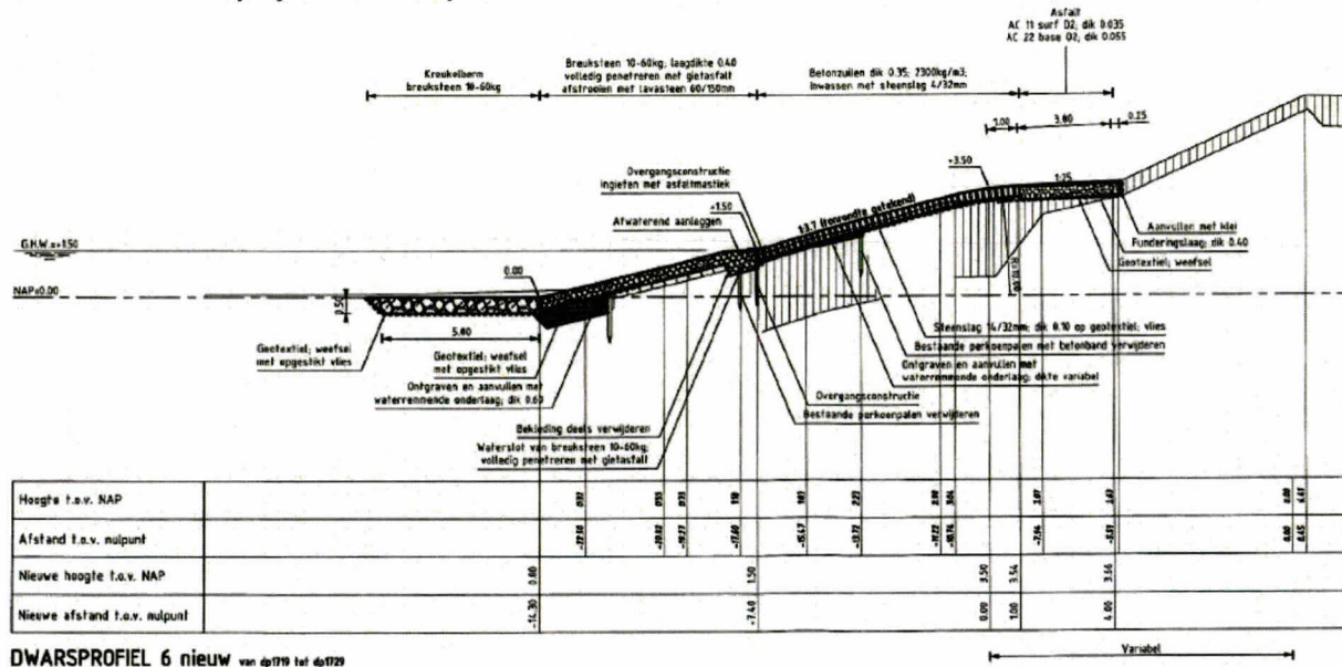
Figuur 2.2: Dwarsprofiel 1, 2, 3, 4, 5 en 6 van de huidige en toekomstige steenbekleding (bron: Van der Vliet, 2012).
