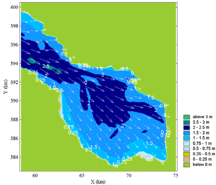
Grid: S3, Wind 300°, Hoog water, 4 m +NAP windsnelheidsklasse 2
