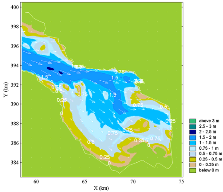
Grid: S3, Wind 300°, Laag water, 0 m +NAP windsnelheidsklasse 2
