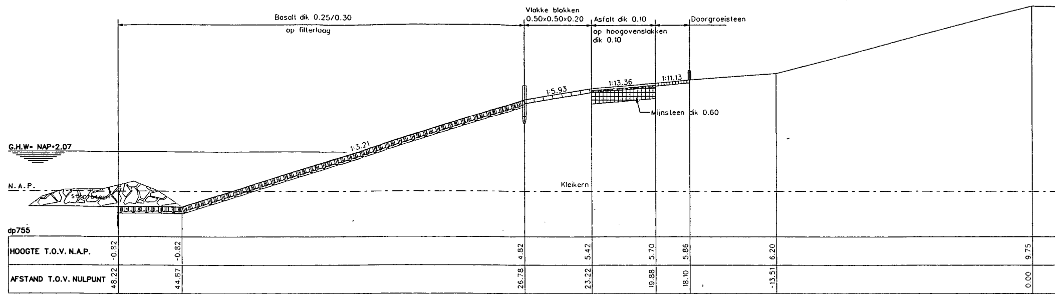
Dwarsprofiel 11 bestaand
