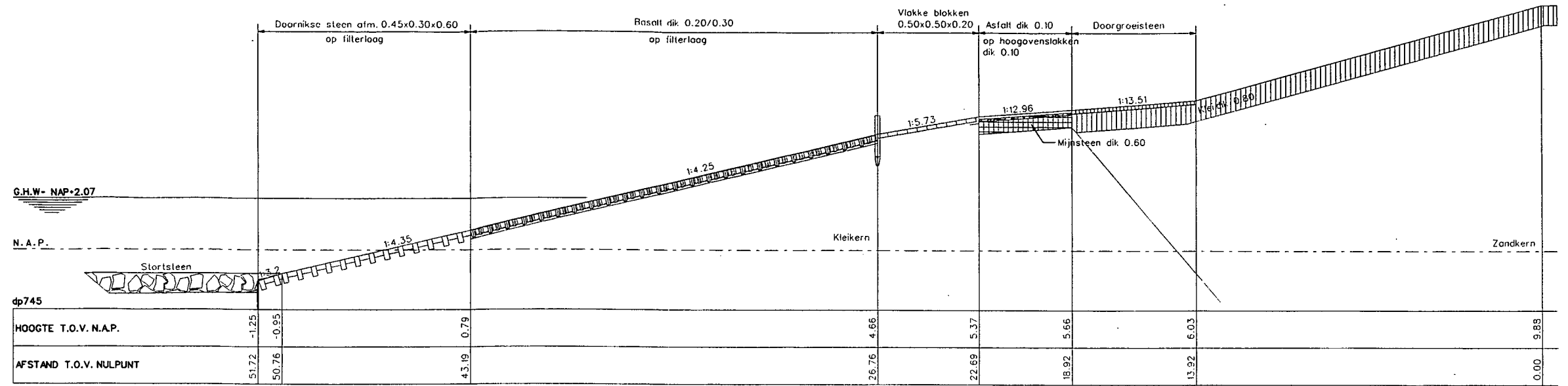
Dwarsprofiel 5 bestaand
