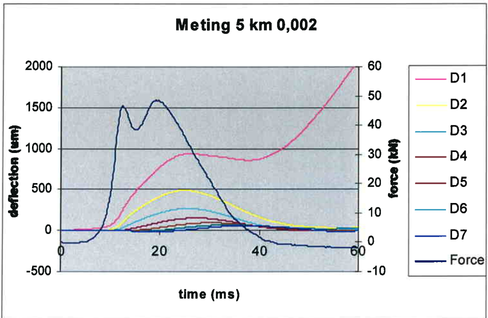
Figuur 3.2: Grafische weergave van de deflectiegolven.
